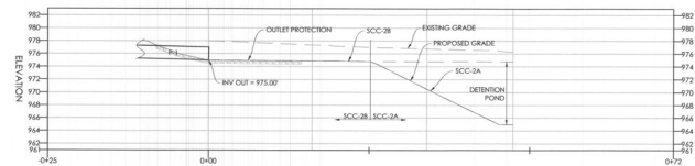
SCC-2A & SCC-2B PROFILE
