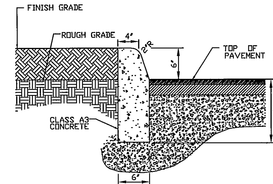
CG-2 DETAIL N.T.S.
