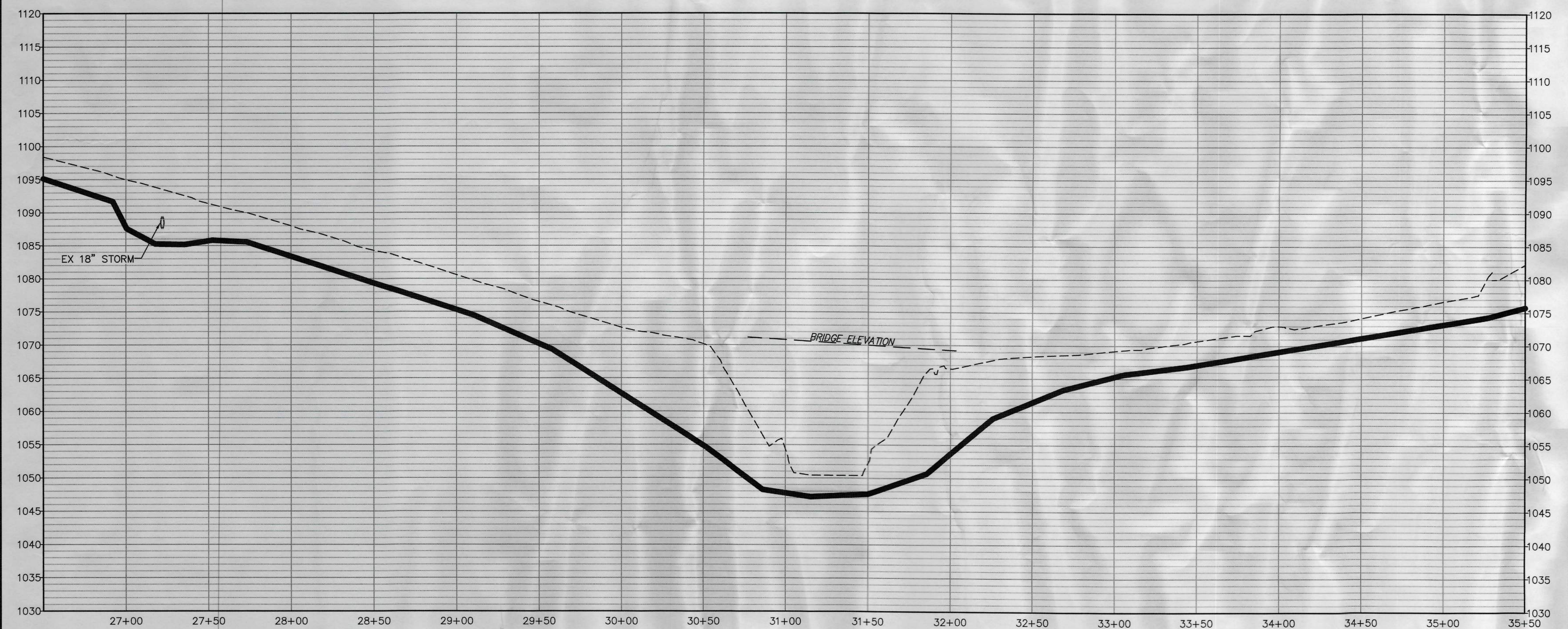
PROFILE: STA 26+50 TO STA 35+50 - Scale: H: 1"=40', V: 1"=10'
