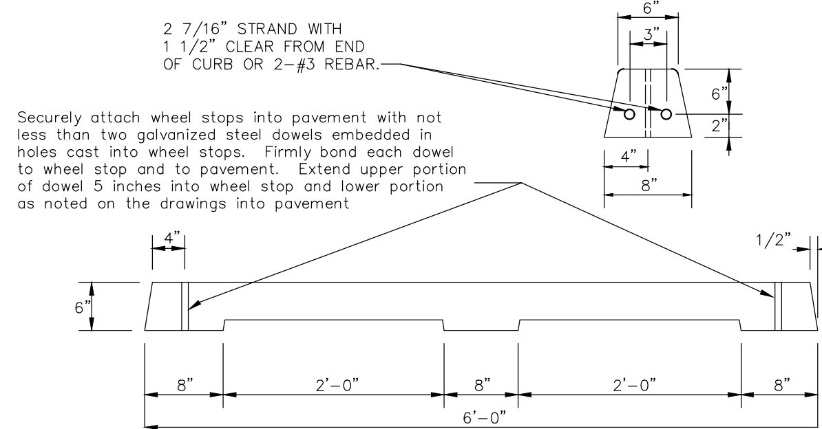
STANDARD WHEEL STOP N.T.S.
