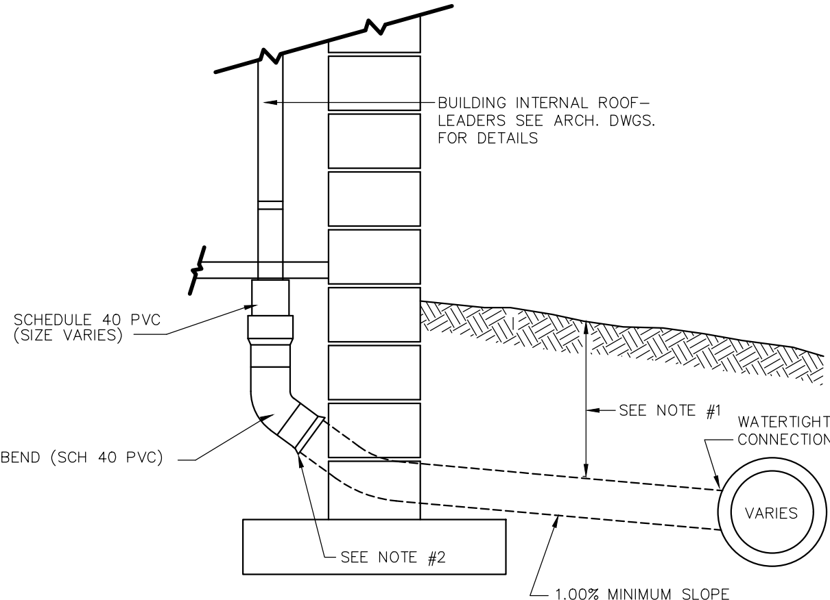
INTERNAL ROOF-LEADER COLLECTOR N.T.S.
