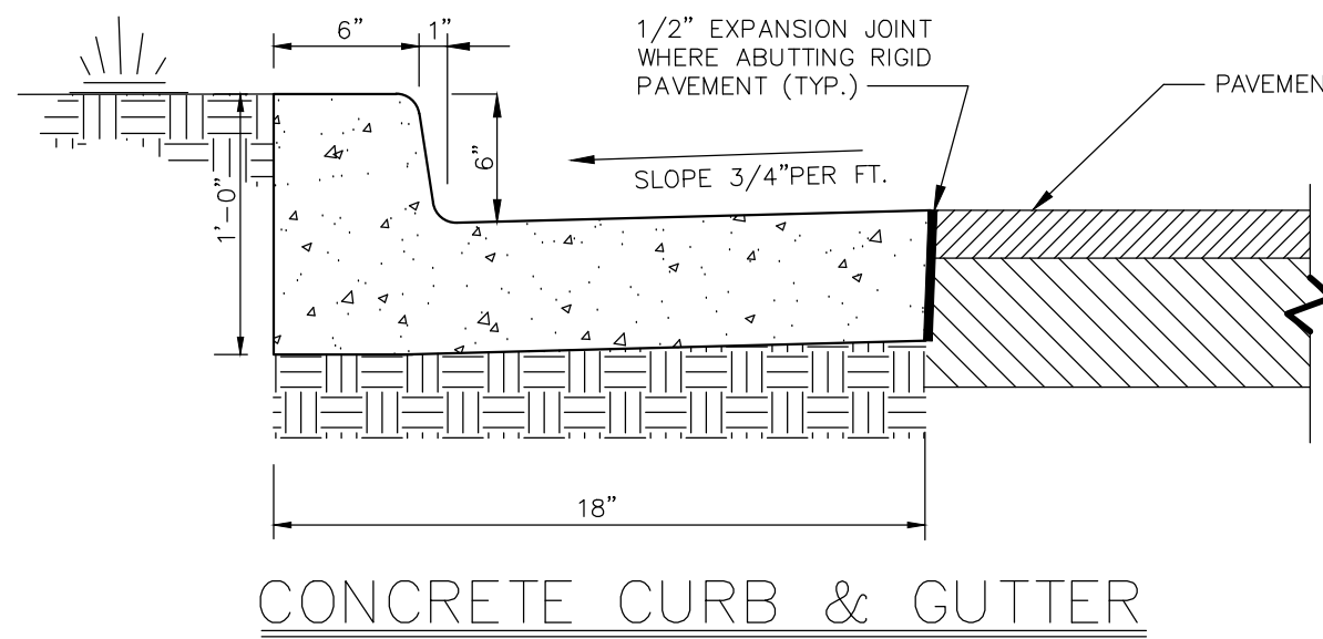
CONCRETE CURB & GUTTER N.T.S.
