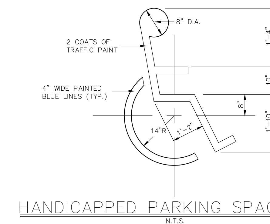
13 DETAIL - HC PARKING SPACE C22.0 SCALE: N.T.S.
