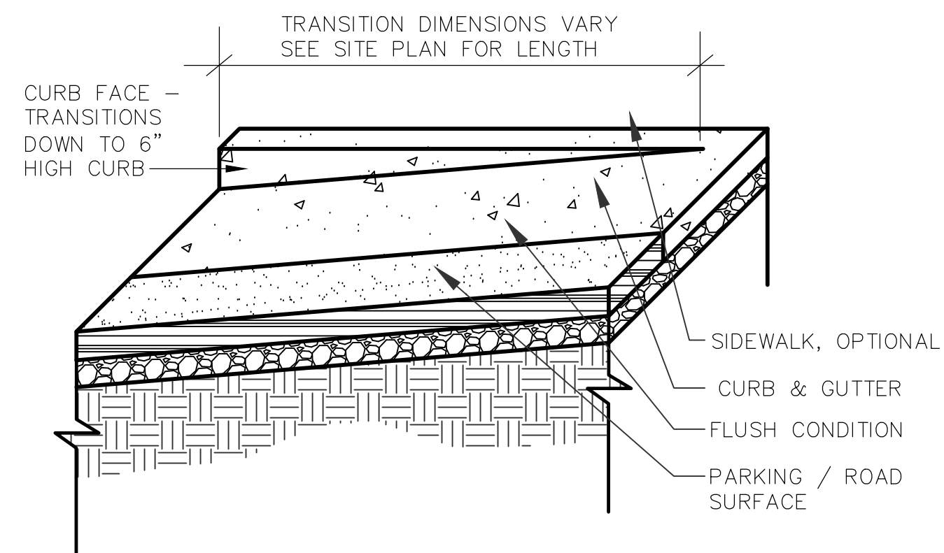
2 TRANSITION CURB DETAIL C22.0 SCALE: N.T.S.
