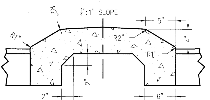
VDOT STD. SI-2
