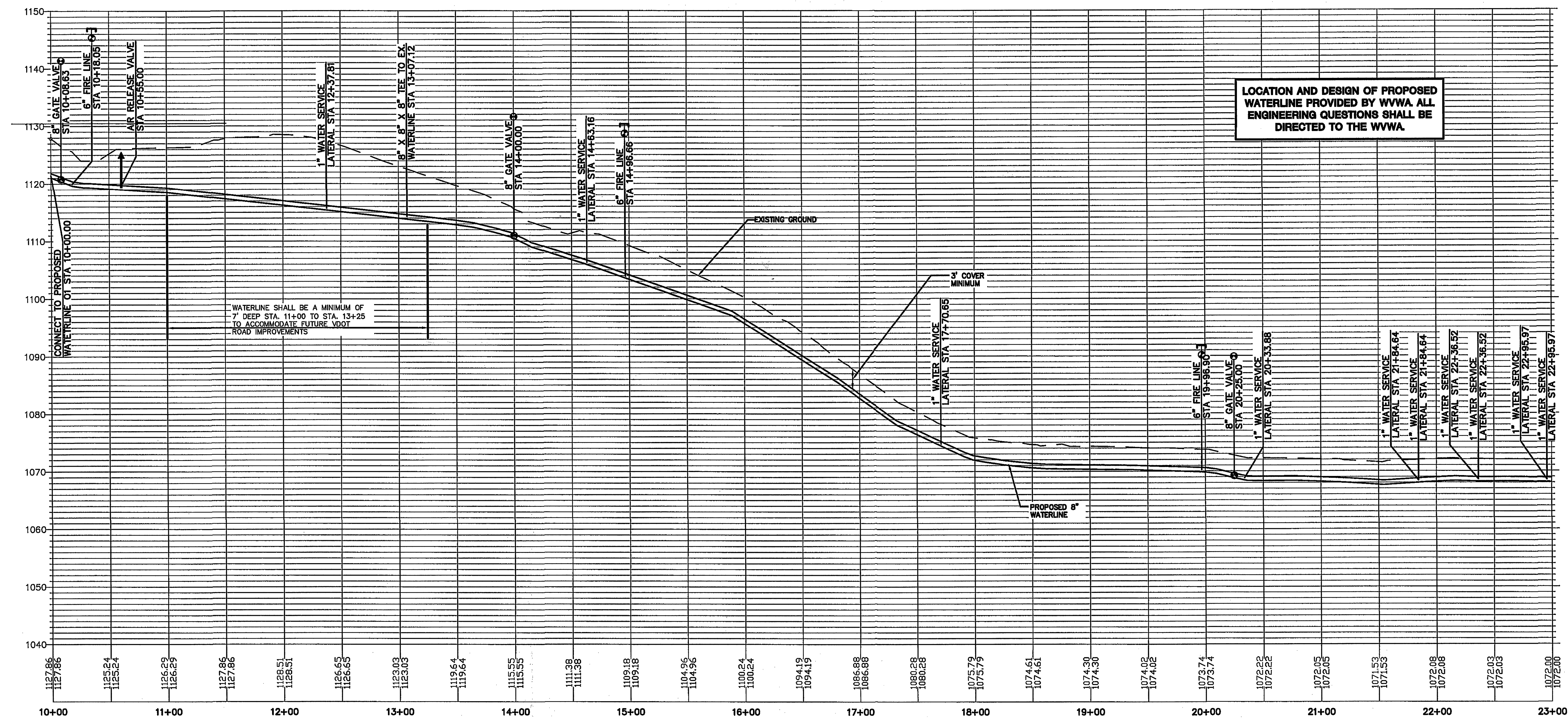
IVYLAND RD. STA 10+00.00 TO STA 23+00.00 PROFILE SCALE: 1"=50'H, 1"=10'V
