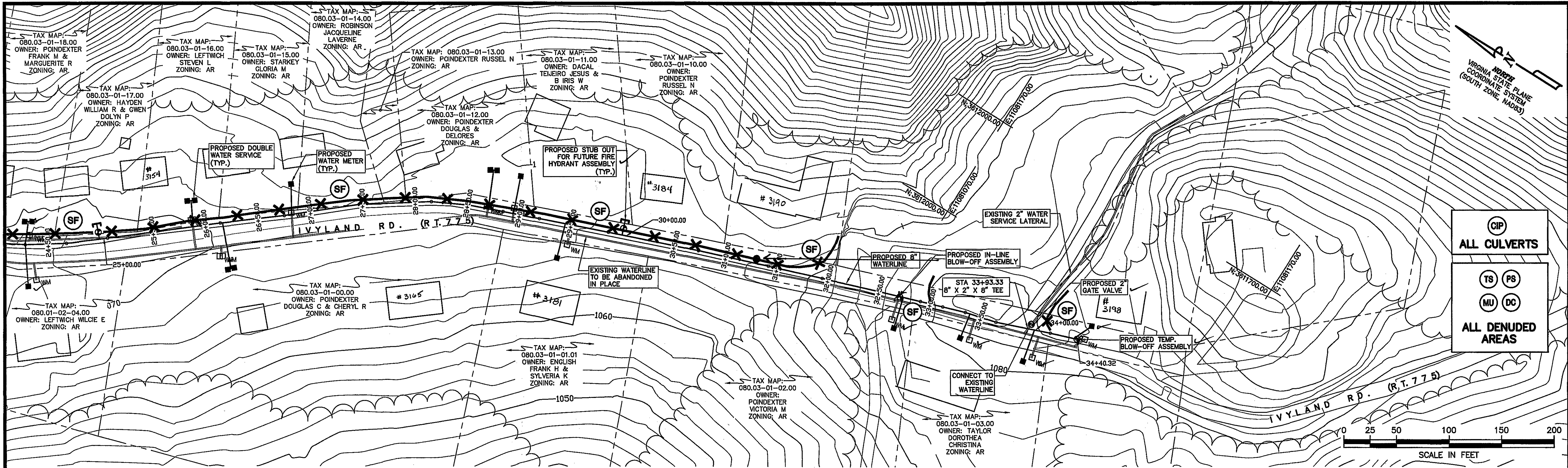
IVYLAND RD. STA 23+00.00 TO STA 34+41.63 PLAN SCALE: 1"=50'
