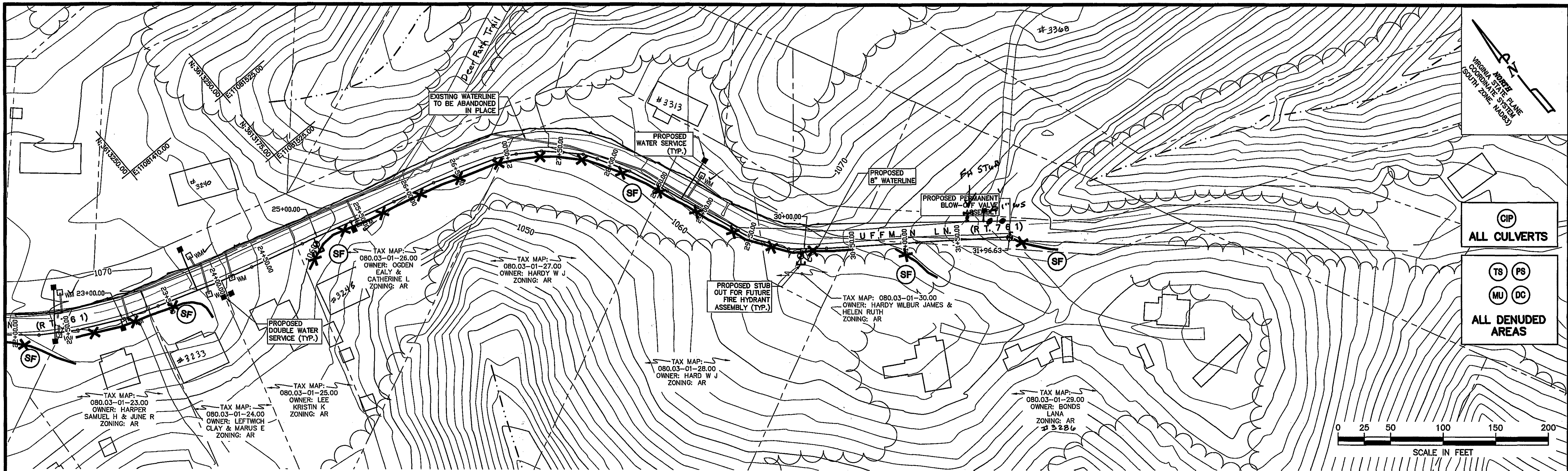
HUFFMAN LN. STA 22+00.00 TO STA 31+96.63 PLAN SCALE: 1"=50'
