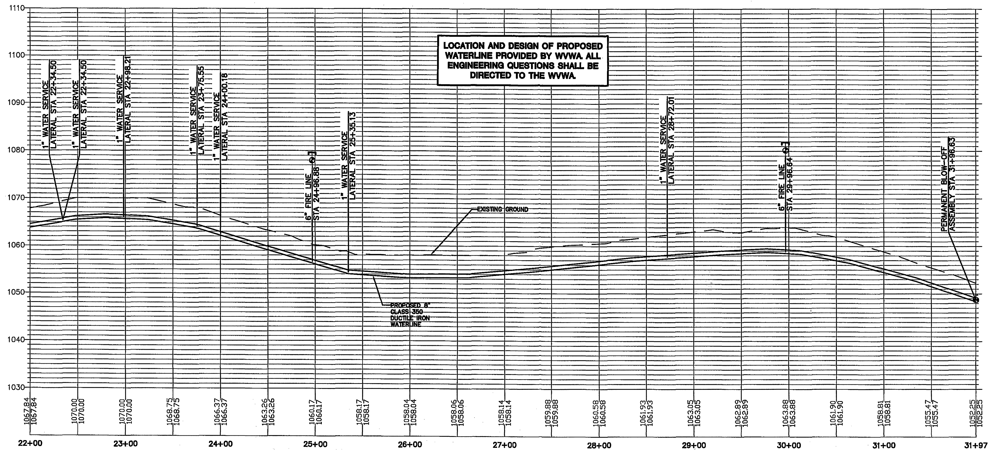
HUFFMAN LN. STA 22+00.00 TO STA 31+96.63 PROFILE SCALE: 1"=50'H, 1"=10'V
