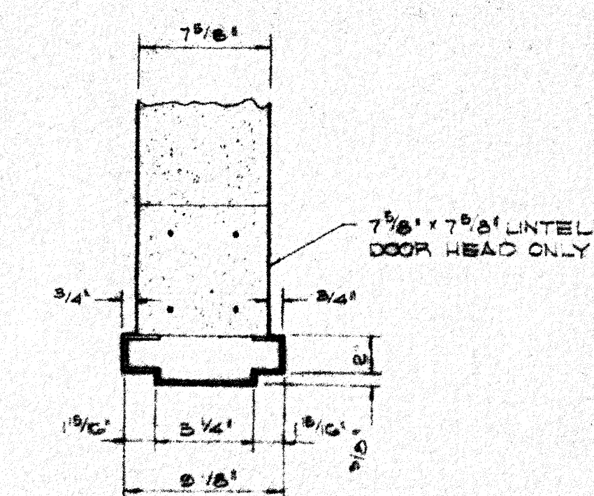
SCALE: 1/2" = 1'-0"
