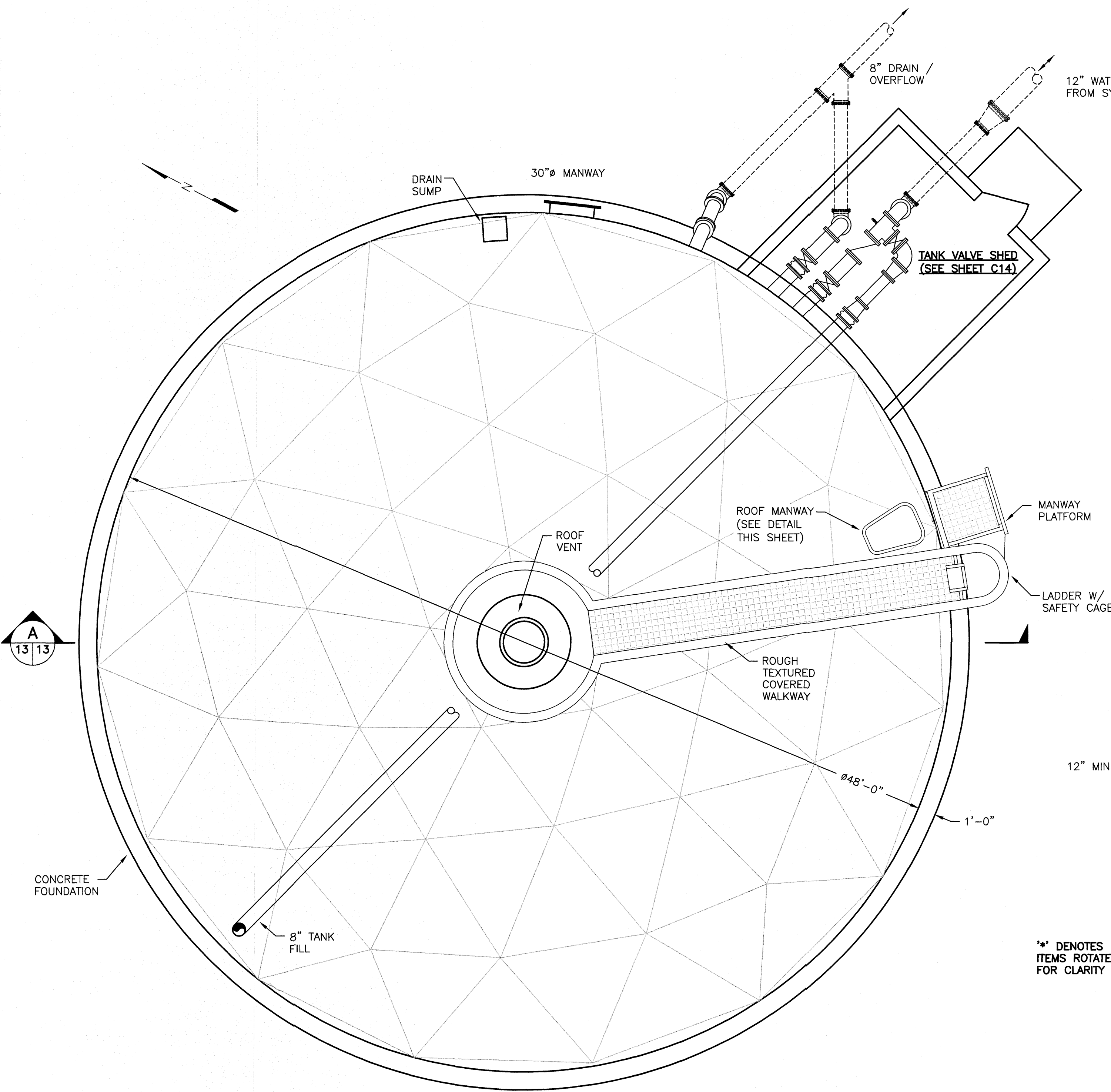
PLAN 1/4"=1'-0"
