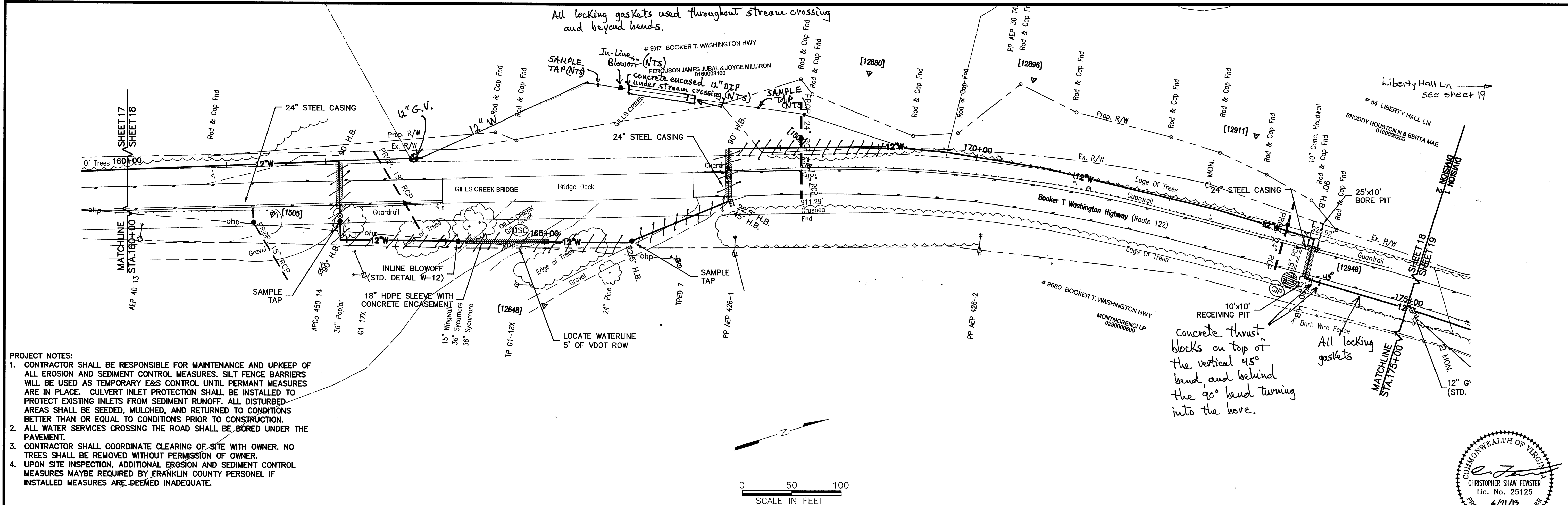
LINE A [STA. 160+00 to STA. 175+00]
