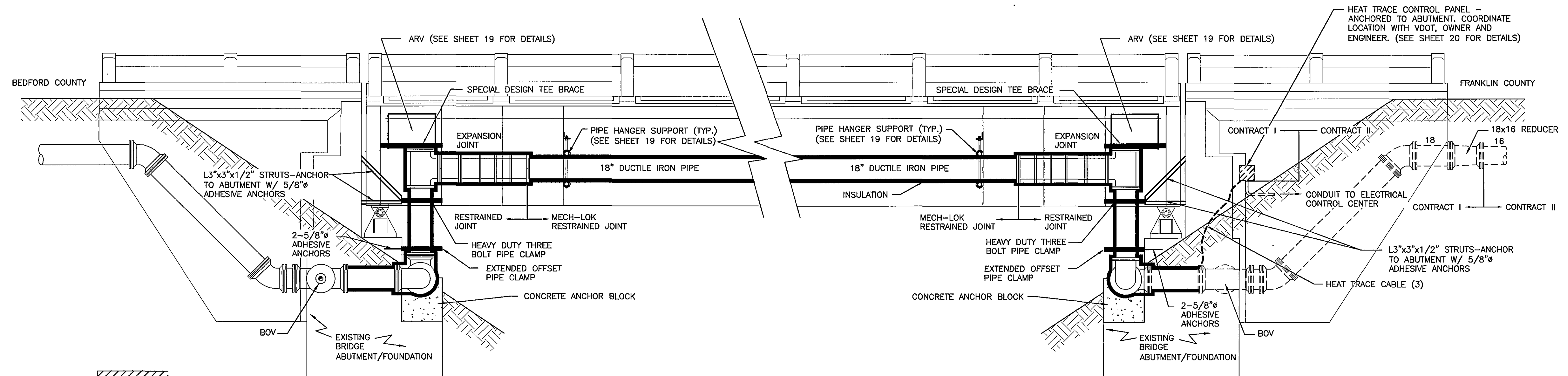
ELEVATION SCALE: 1/4" = 1'-0"
