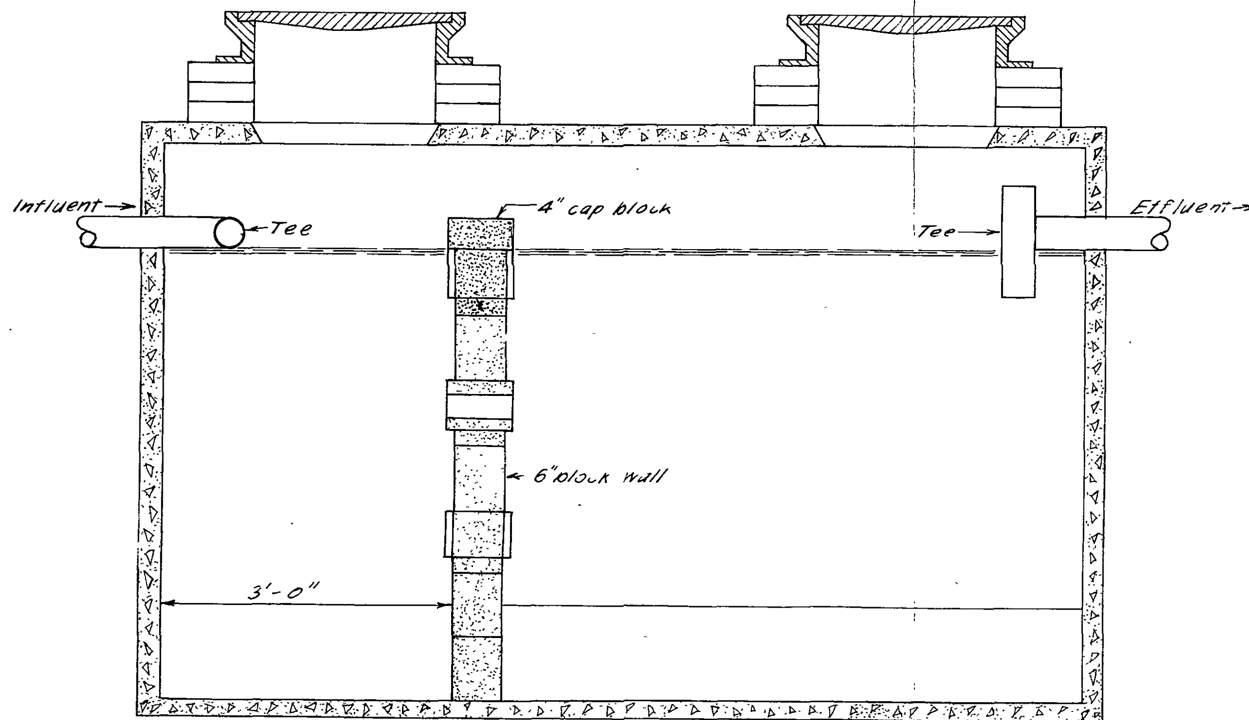
SECTION A--A' Scale: 1 inch = 1 foot
