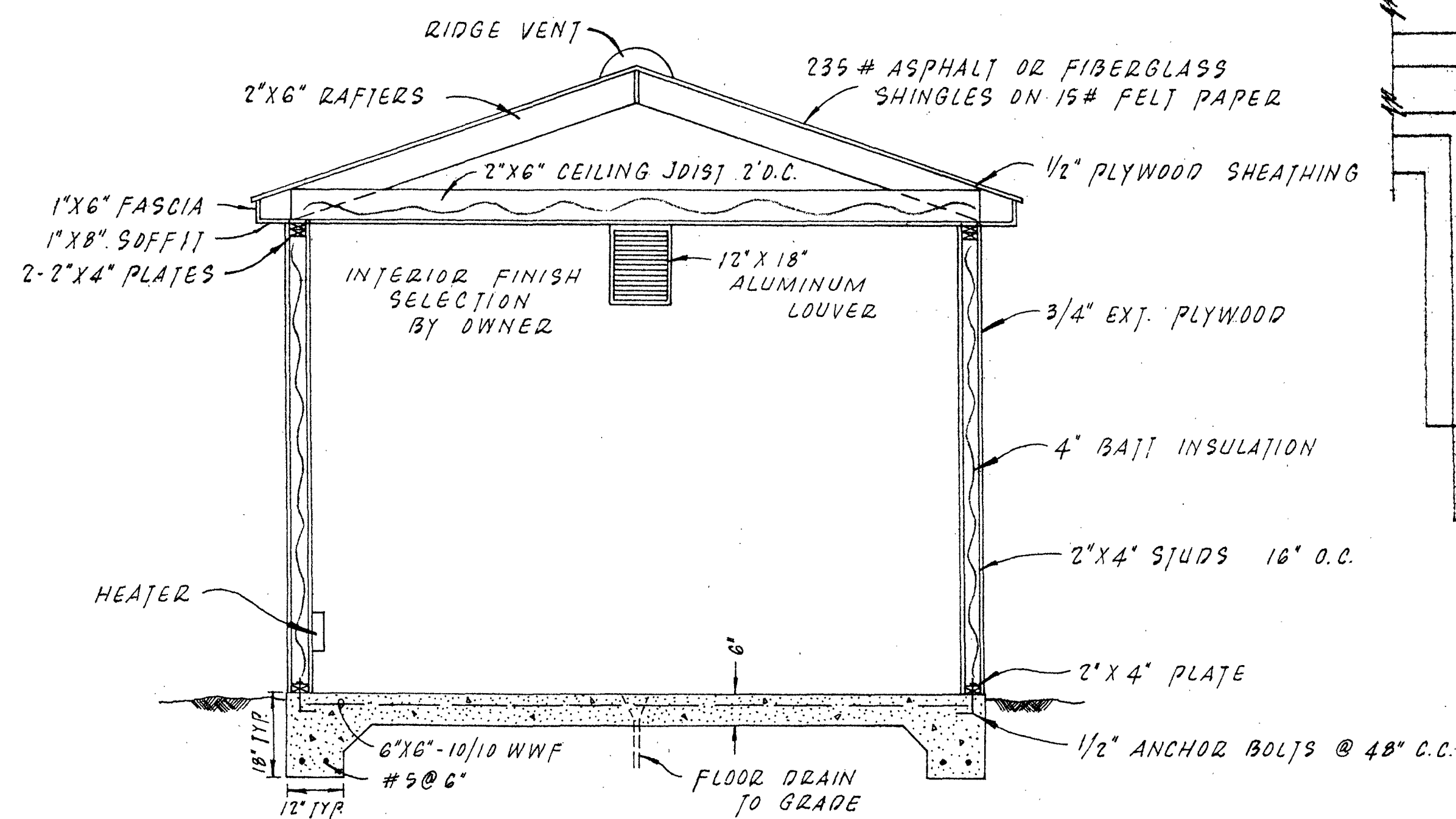
SECTION A-A
