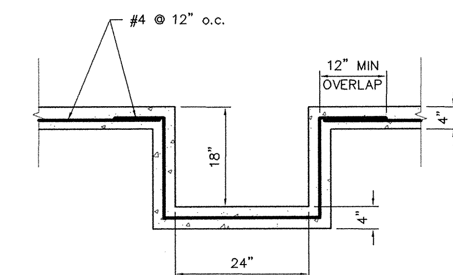
2 TRENCH DRAIN SECTION SCALE: 3/4" = 1'-0"
