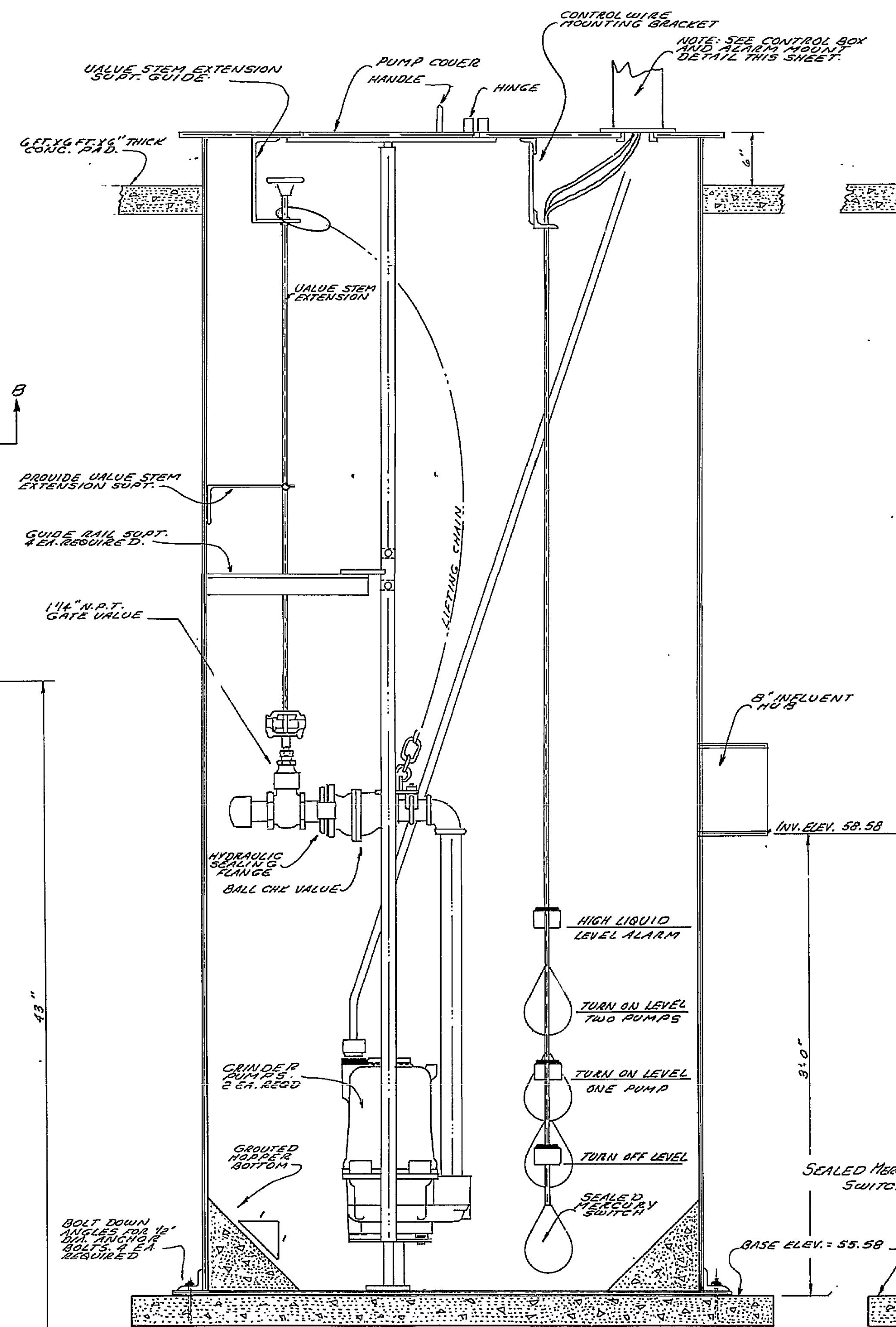
SECTION A-A
