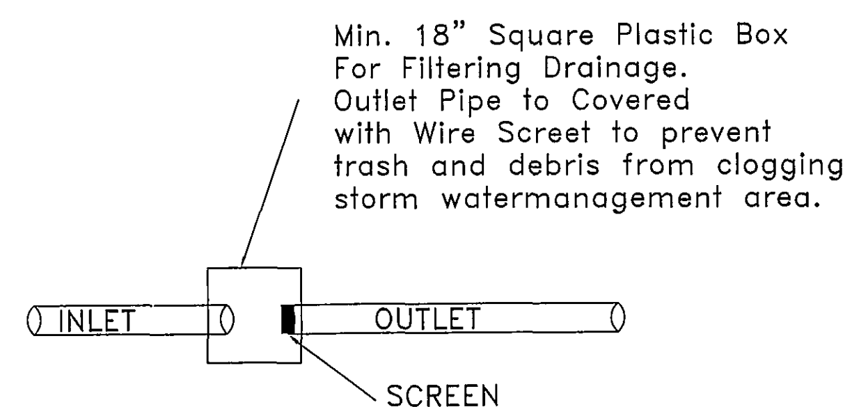
FITLER BOX DETAIL N.T.S.
