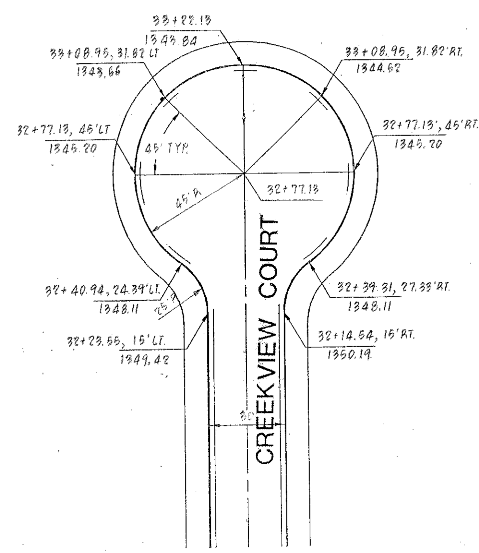
CUL-DE-SAC
