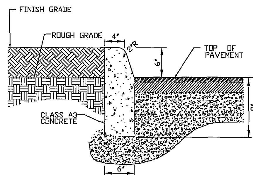
CG-2 DETAIL TYP. N.T.S.
