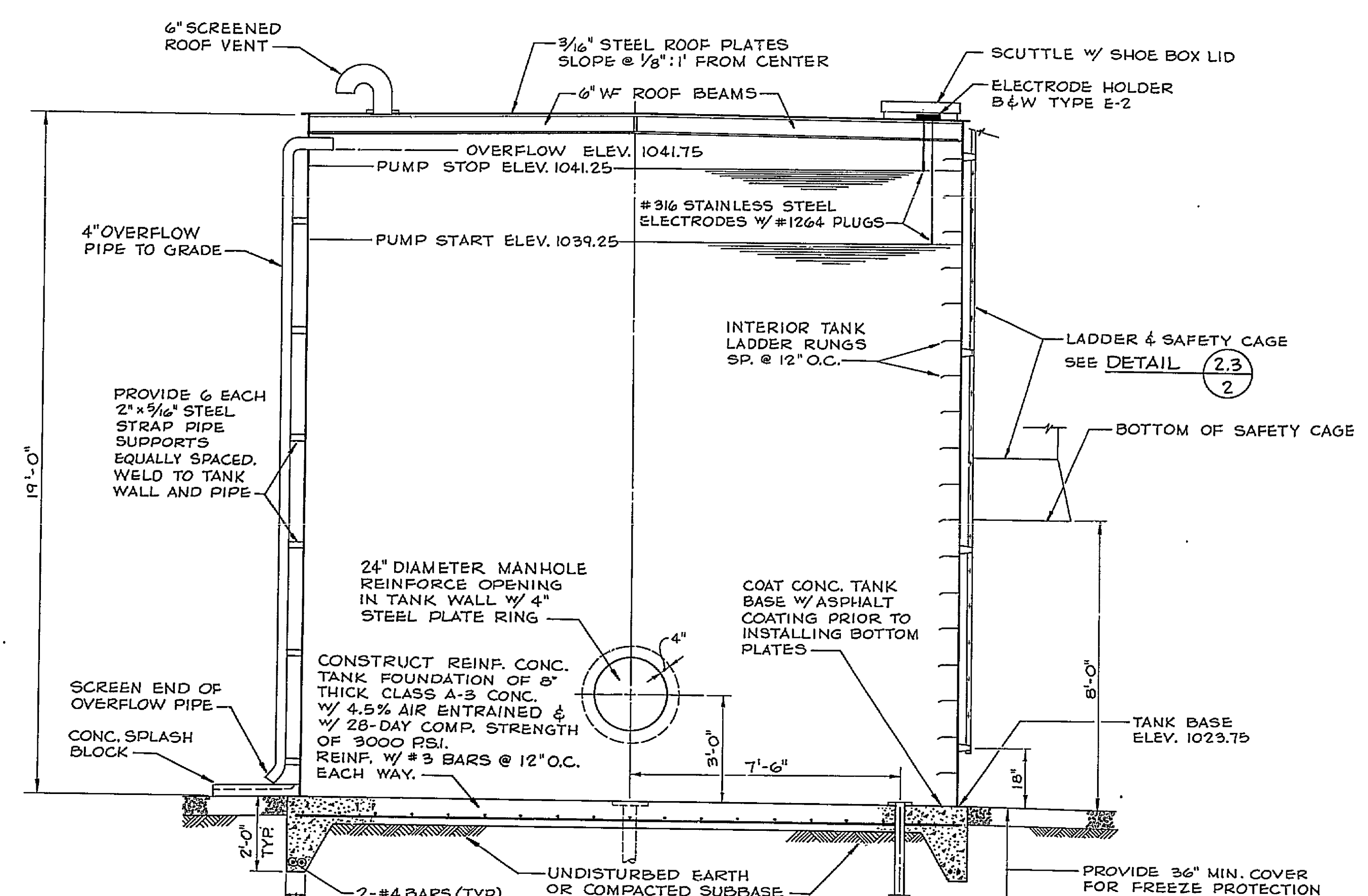
SECTION 2.1 SCALE: \frac{3}{8}" = 1'-0"
