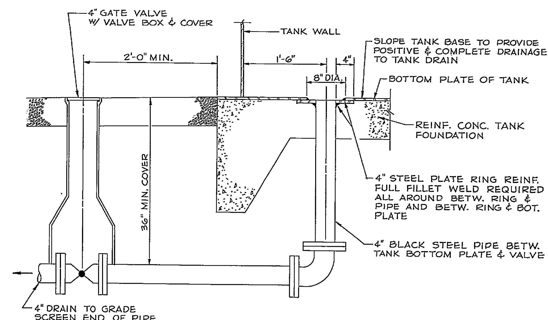
SECTION 2.5 SCALE: 1"=1'-0"
