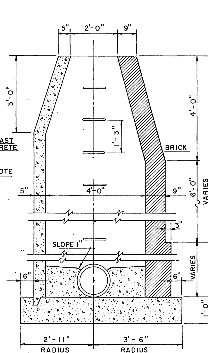
LONGITUDINAL SECTION
