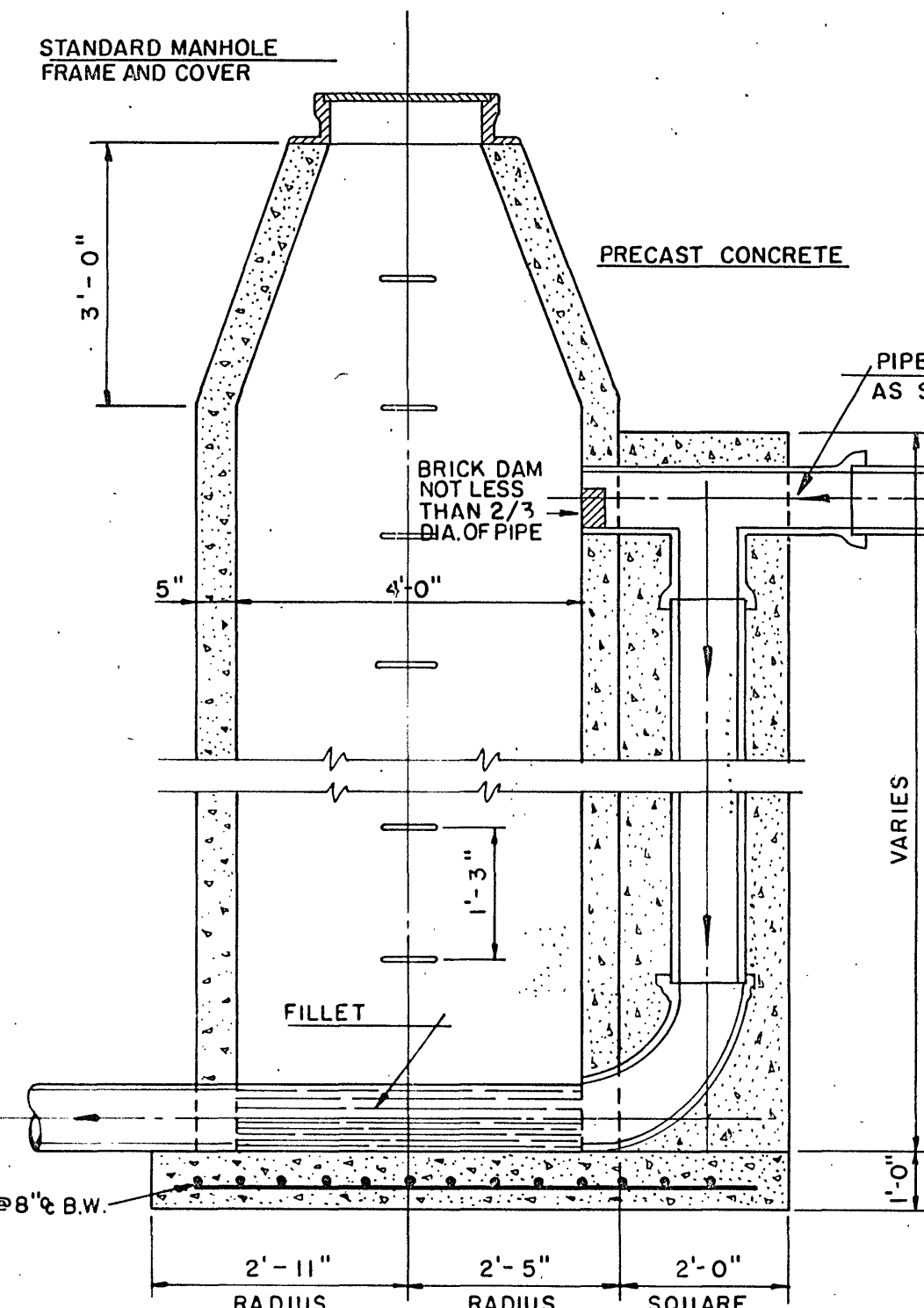
LONGITUDINAL SECTION
