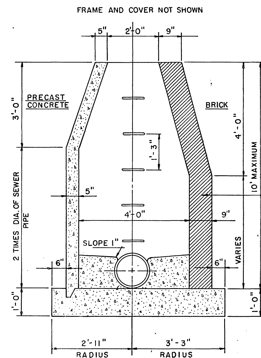
LONGITUDINAL SECTION
