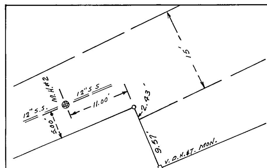
INSERT DETAIL SCALE: 1" = 5'
