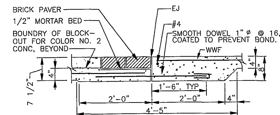
BRICK SECTION A6.15 SCALE: 3/4" = 1'-0" A1
