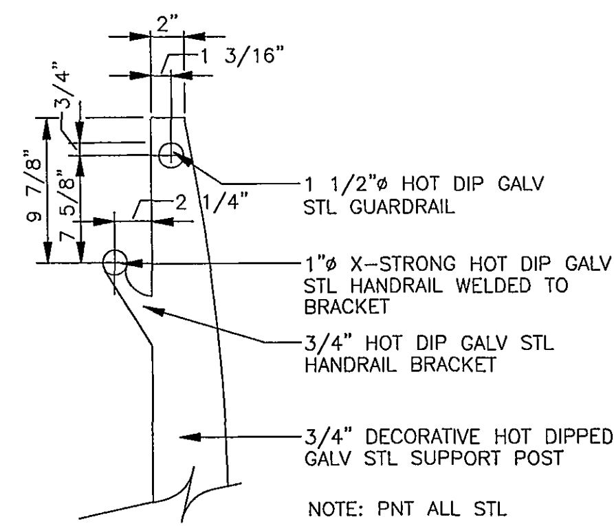
HANDRAIL DETAIL A6.2 SCALE: 1 1/2" = 1'-0" A5
