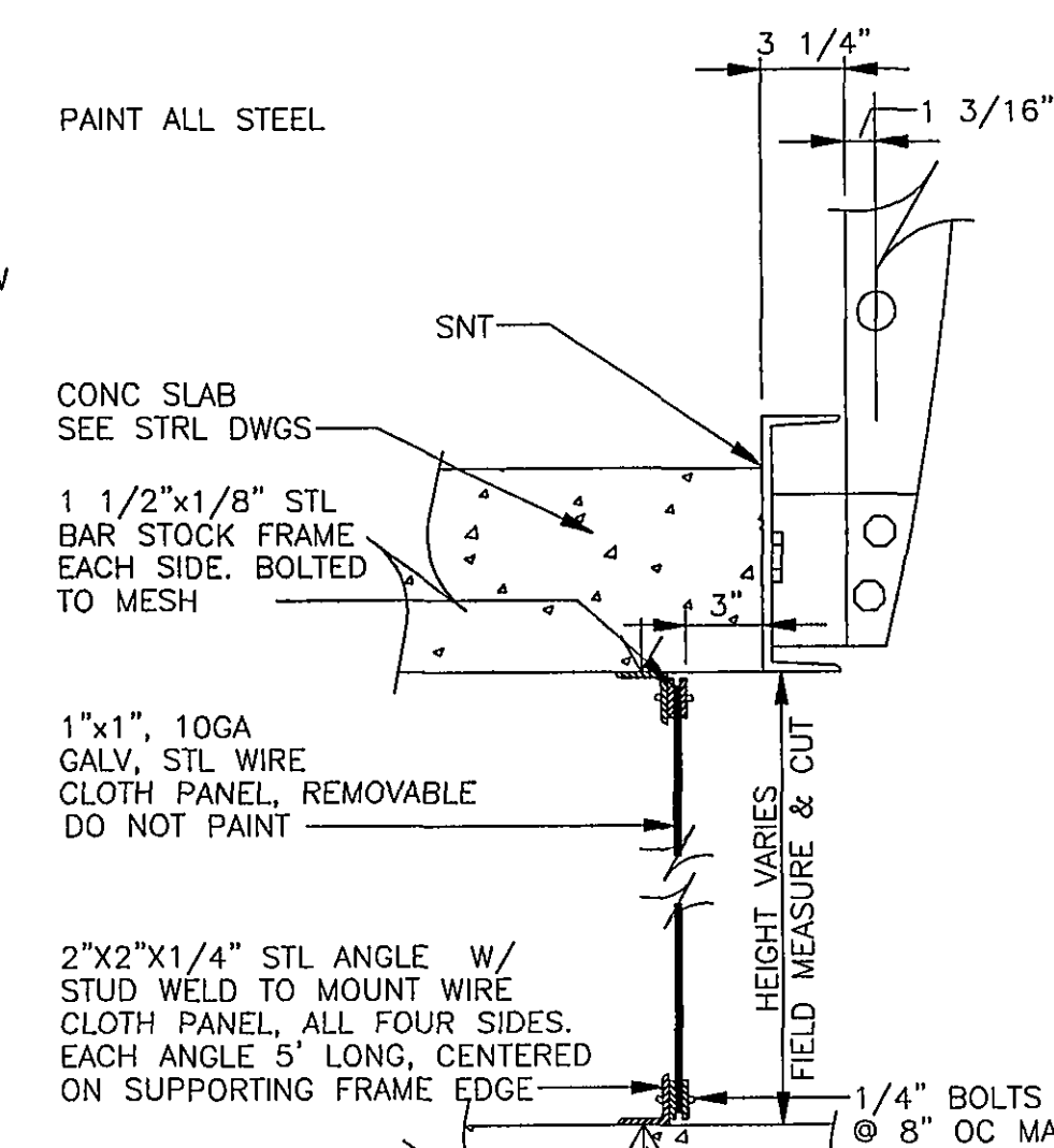
GUARDRAIL DETAIL A6.3 SCALE: 1 1/2" = 1'-0" A5
