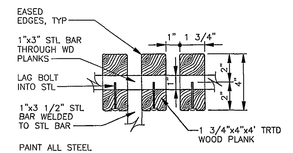
BENCH DETAIL A6.10 SCALE: 3" = 1'-0" A2
