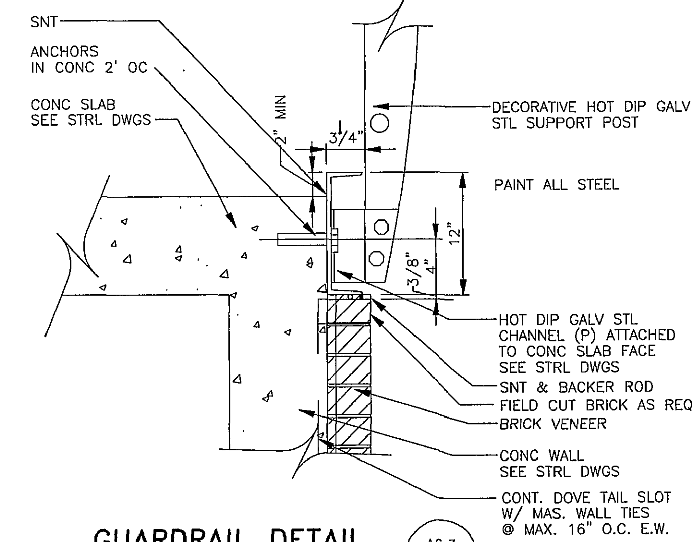
GUARDRAIL DETAIL A6.3 SCALE: 1 1/2" = 1'-0" A5
