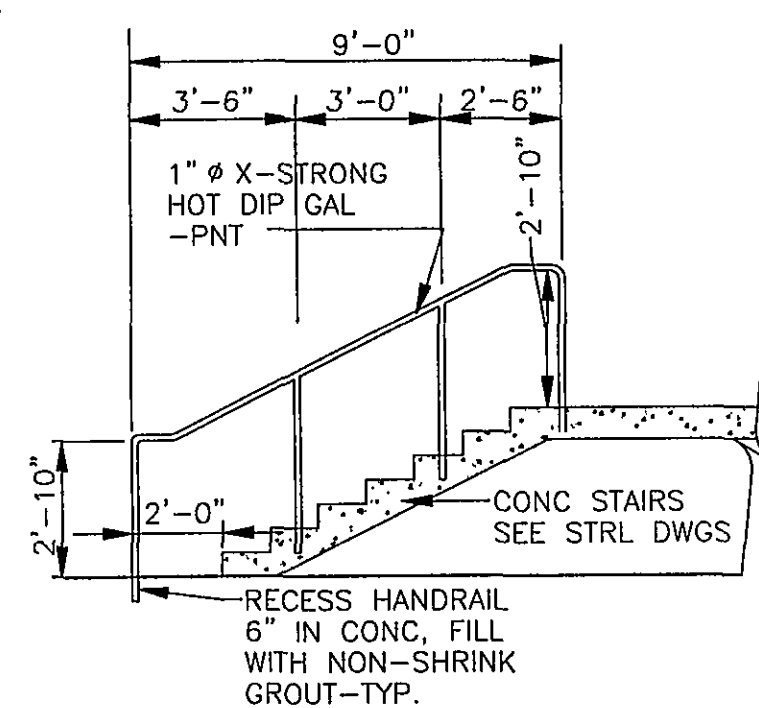
DETAIL A6.11 SCALE: 1/4" = 1'-0" A4
