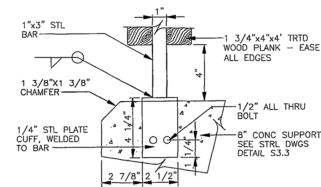
BENCH DETAIL A6.9 SCALE: 3" = 1'-0" A2
