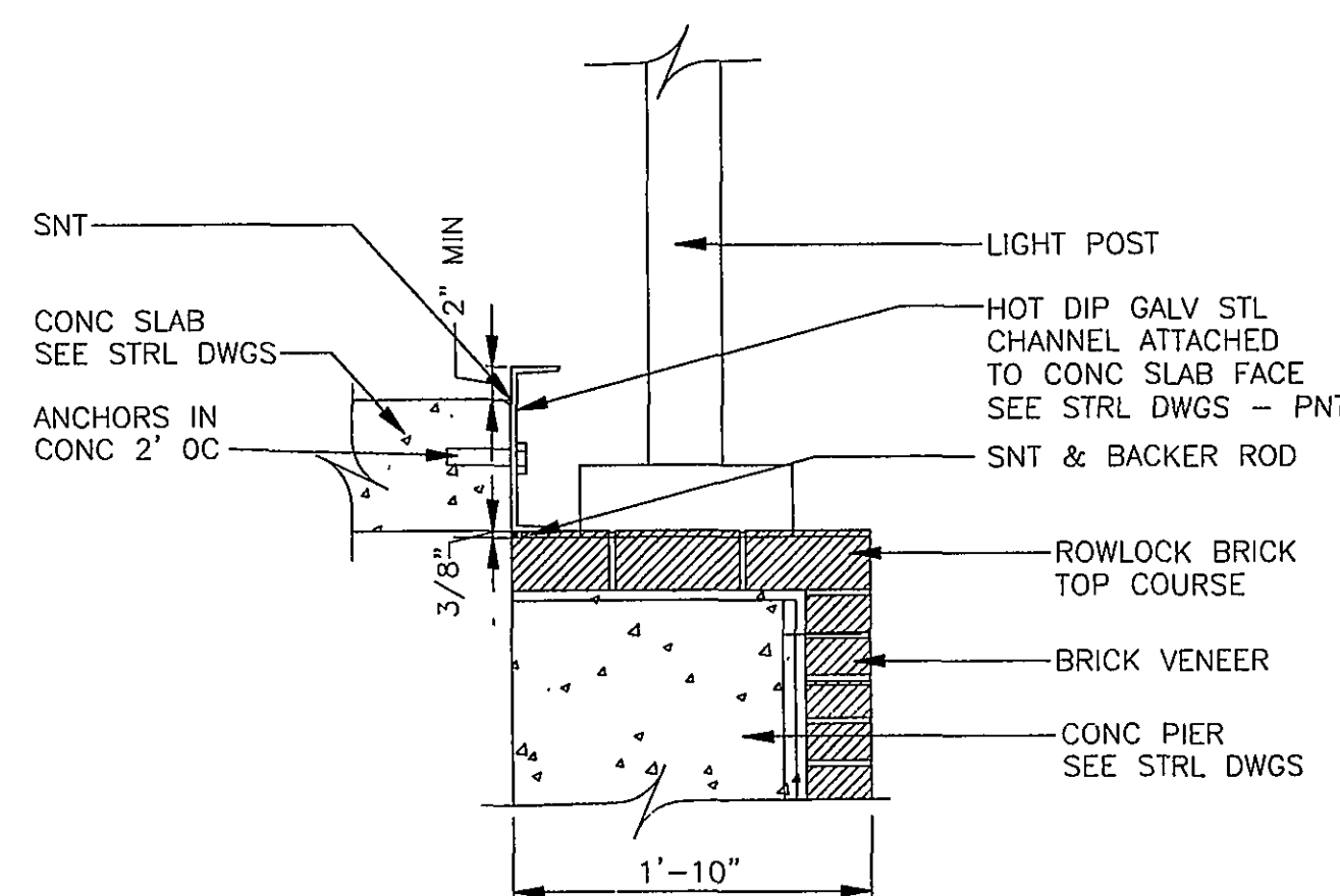
DETAIL A6.13 SCALE: 1/4" = 1'-0" A5
