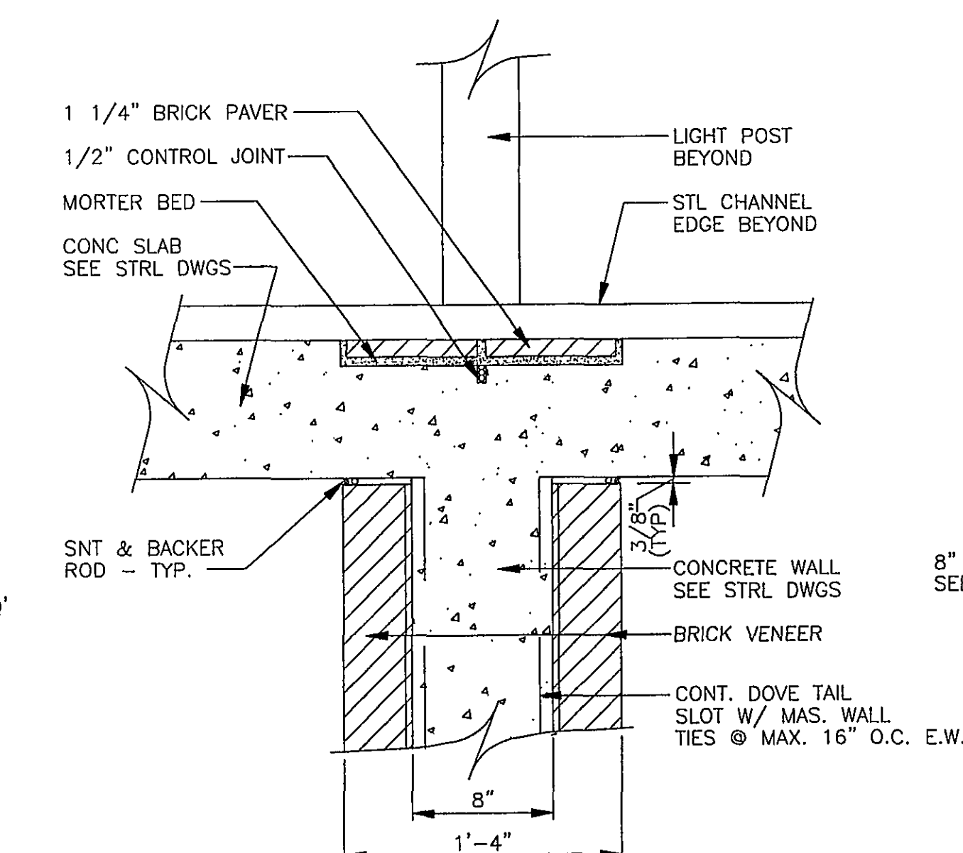
BRICK PAVER DETAIL A6.4 SCALE: 1 1/2" = 1'-0" A5
