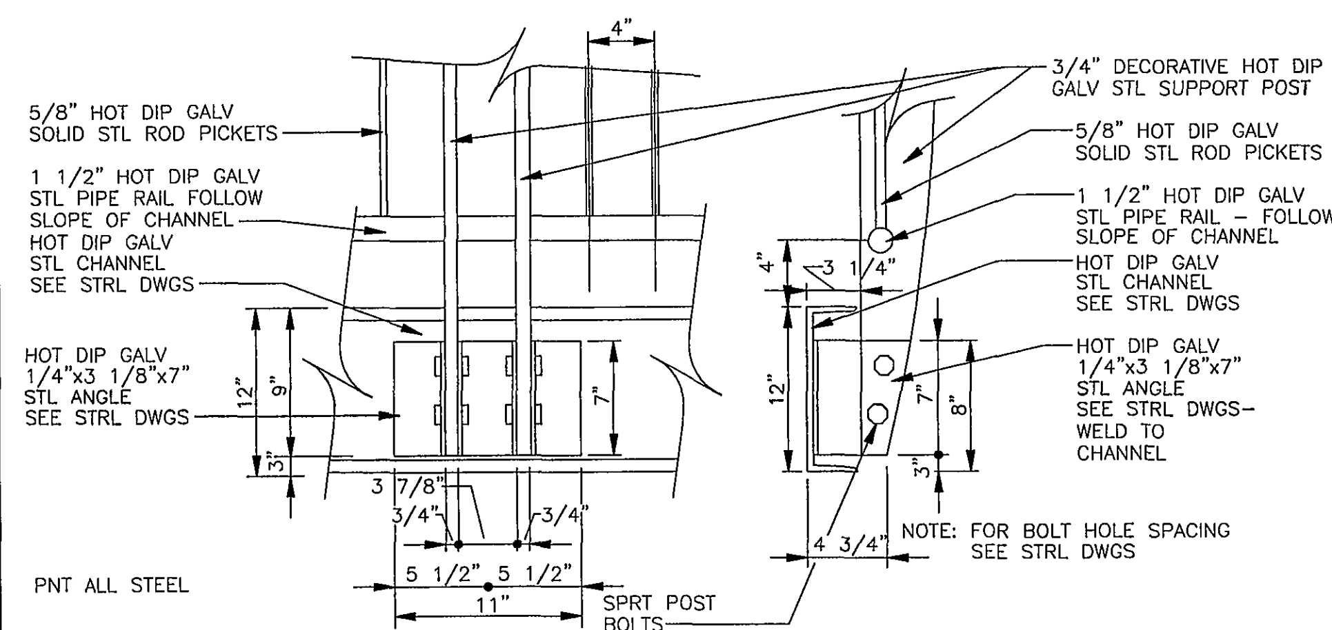
GUARDRAIL DETAIL A6.6 SCALE: 1 1/2" = 1'-0" A5
