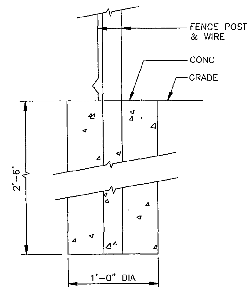
FTG DETAIL A6.12 SCALE: 1 1/2" = 1'-0" A2
