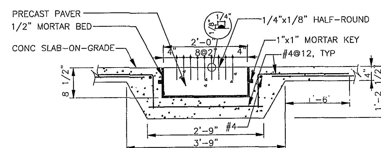
PRECAST SECTION A6.14 SCALE: 3/4" = 1'-0" A1
