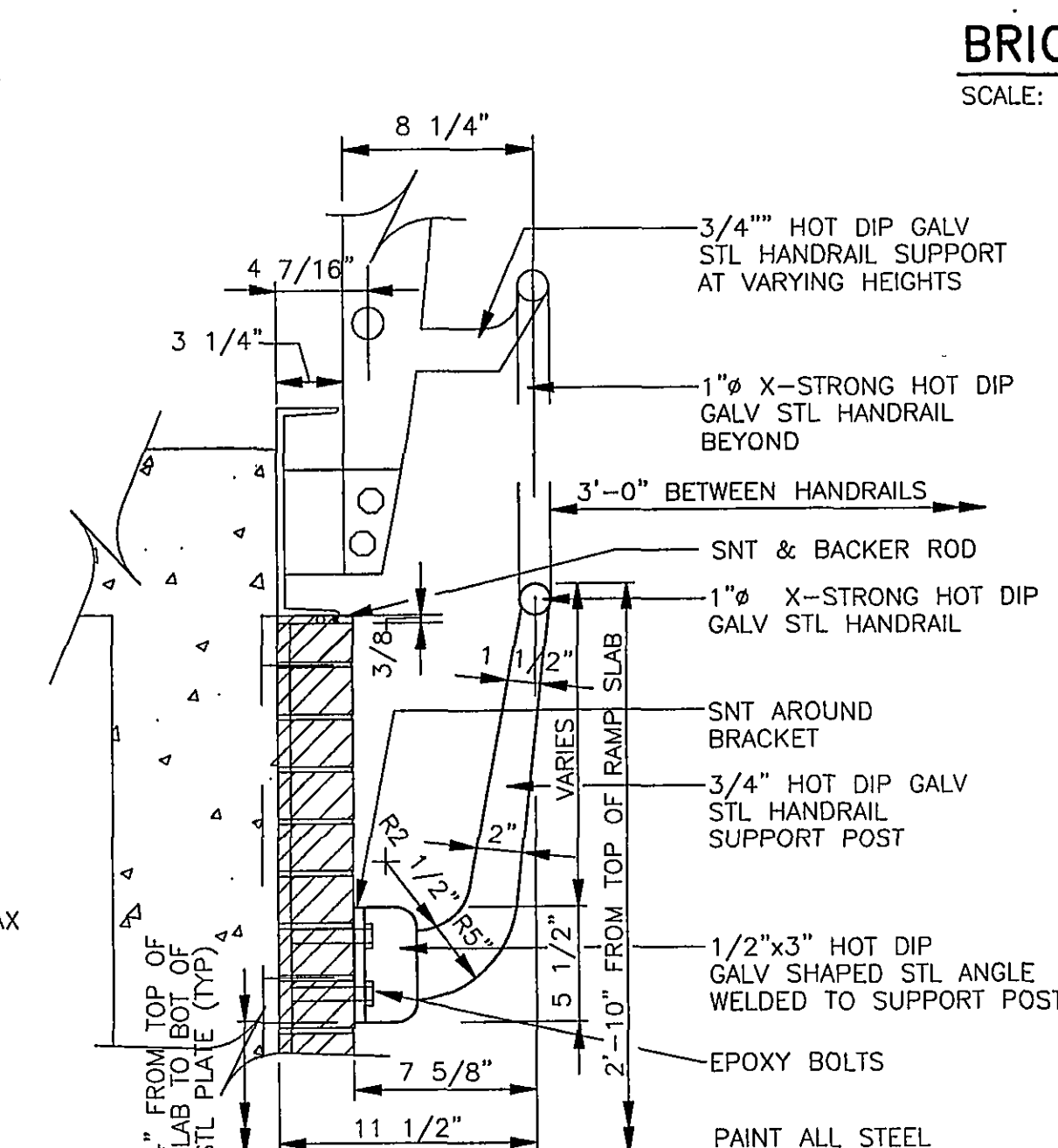
GUARDRAIL DETAIL A6.3 SCALE: 1 1/2" = 1'-0" A5
