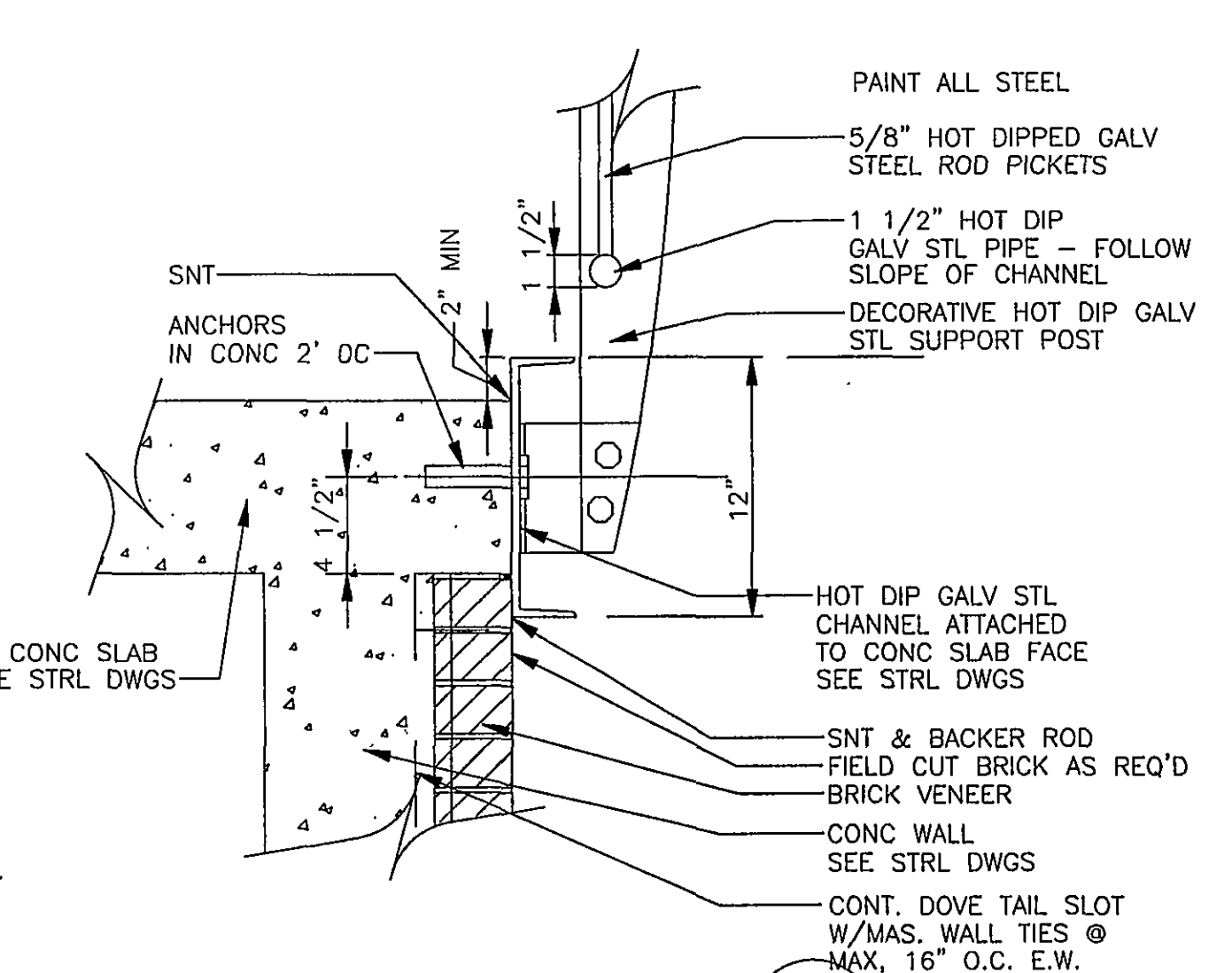
GUARDRAIL DETAIL A6.5 SCALE: 1 1/2" = 1'-0" A1 A5
