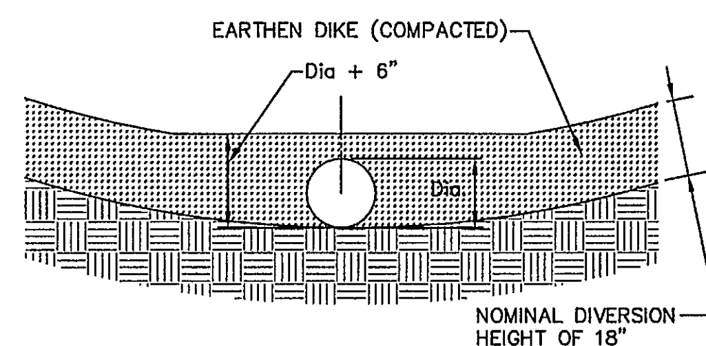
SECTION A-A
