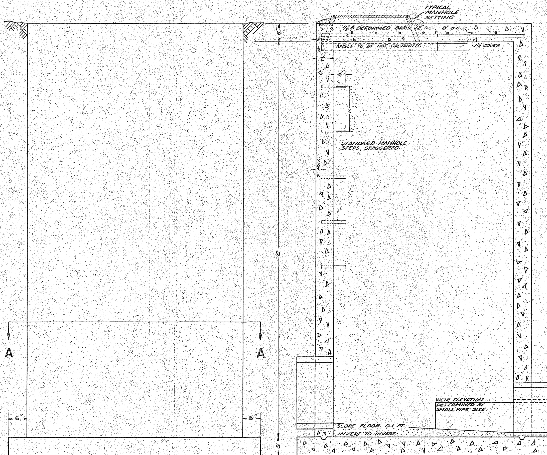
ELEVATION
