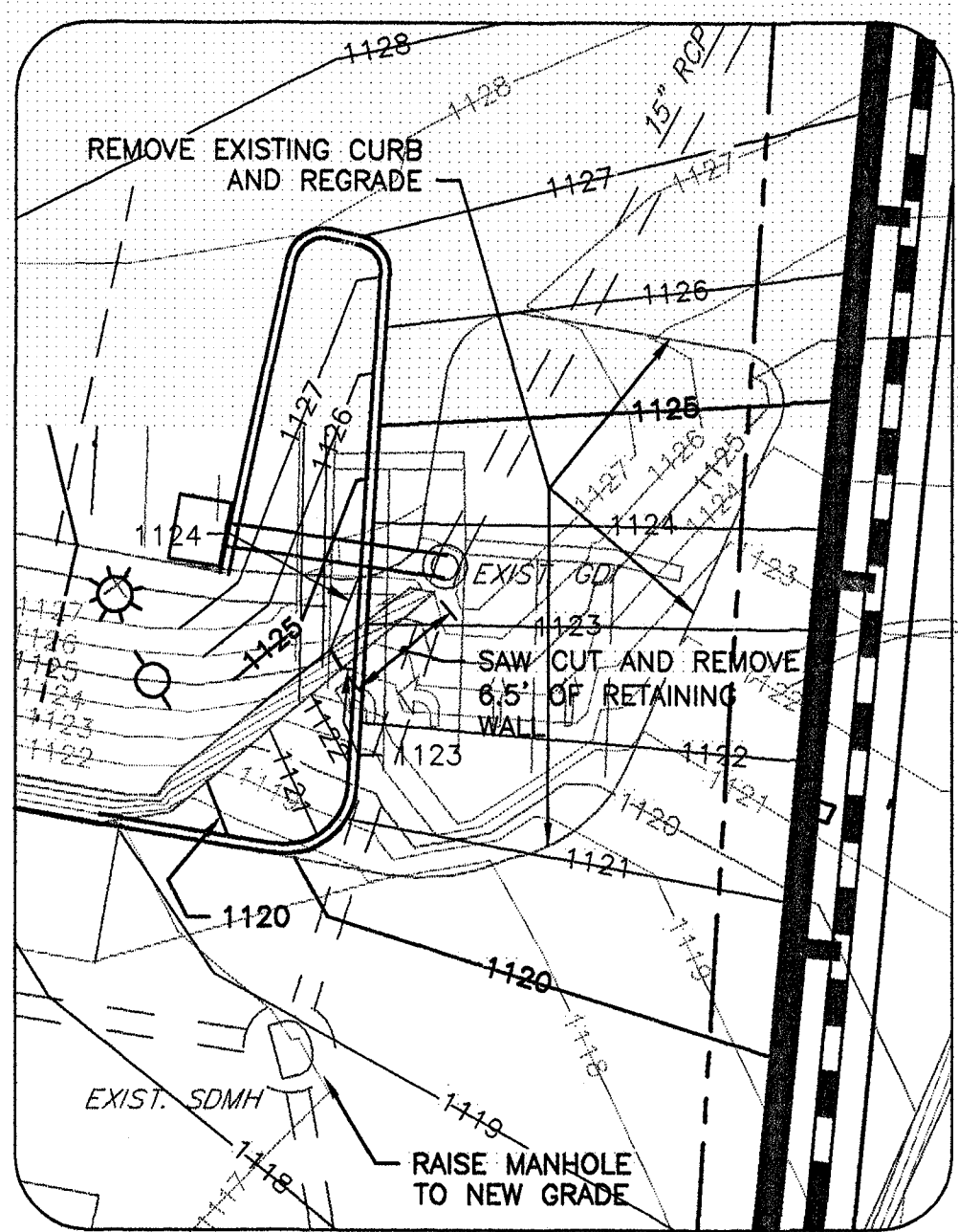
DETAIL (SCALE: 1"=10')
