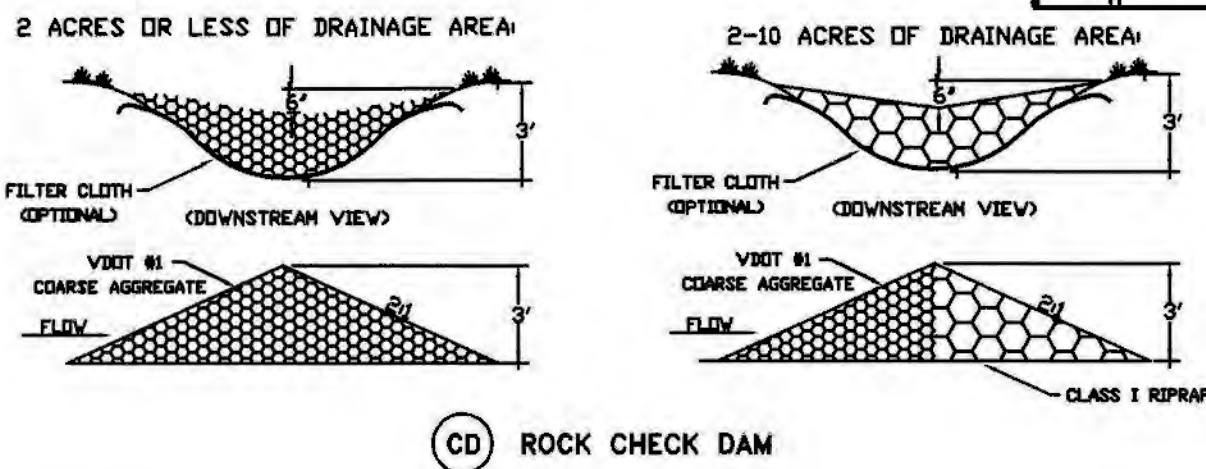
(CD) ROCK CHECK DAM
