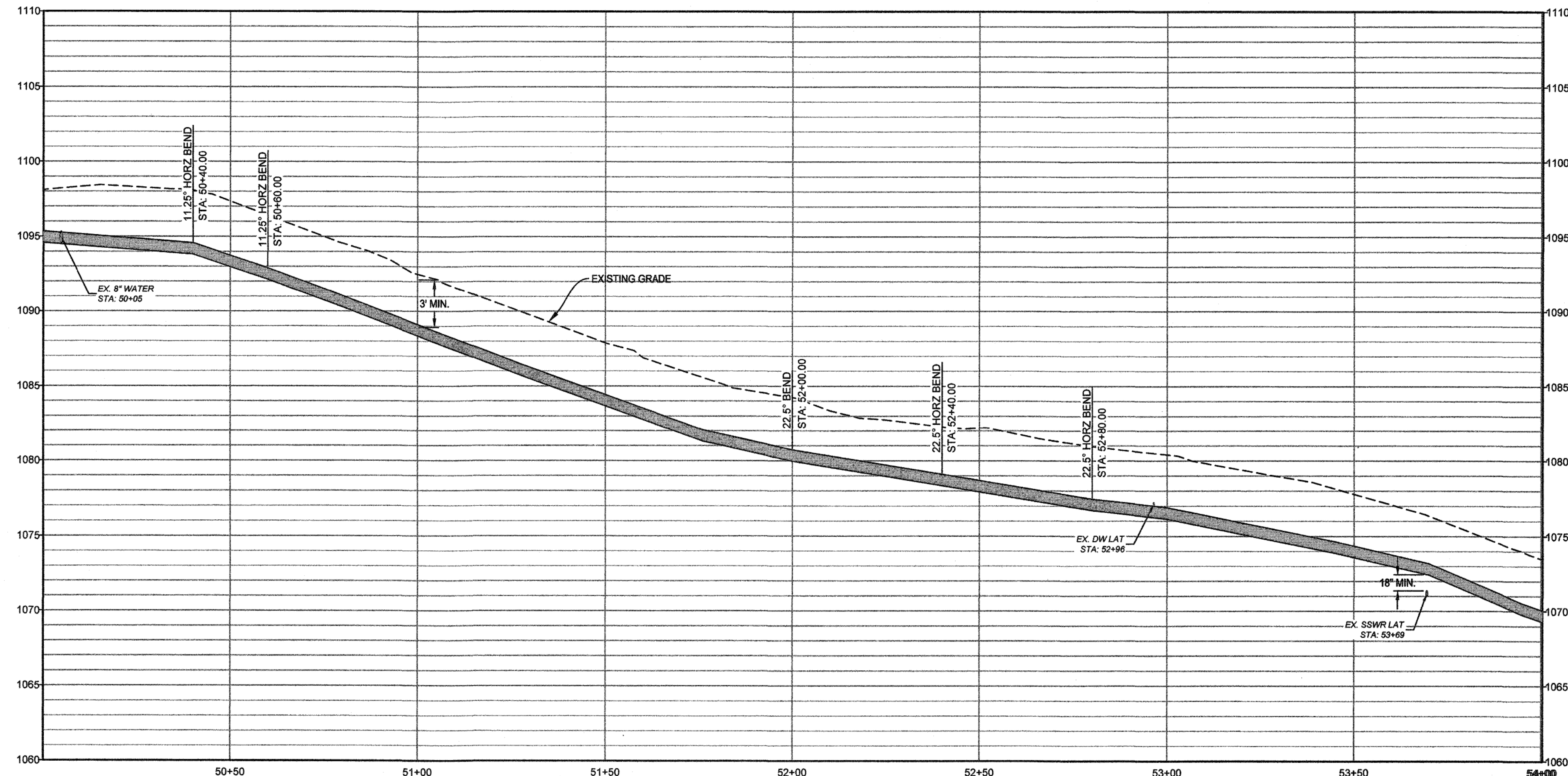
PROFILE: STA 50+00 TO STA 54+00 - Scale: H: 1"=20', V: 1"=5'
