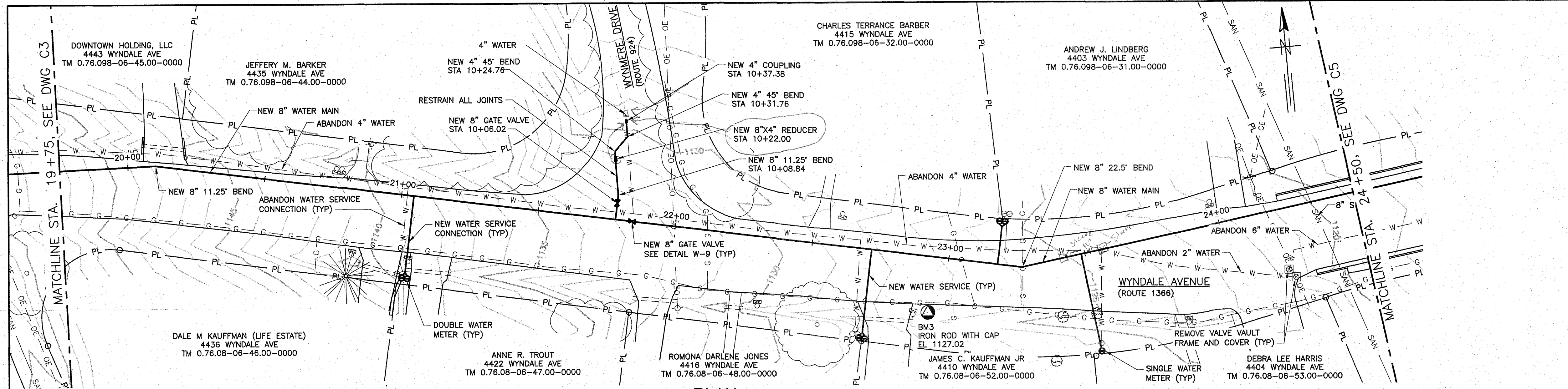
PLAN SCALE: 1" = 20'
