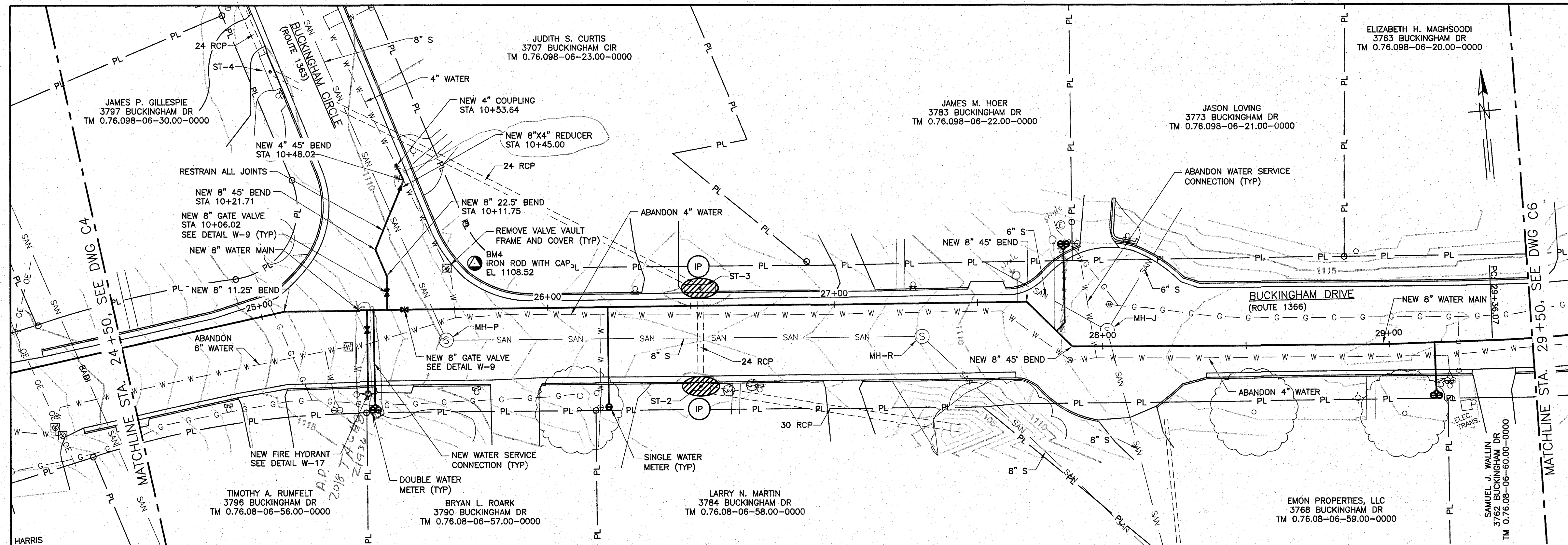
PLAN SCALE: 1" = 20'
