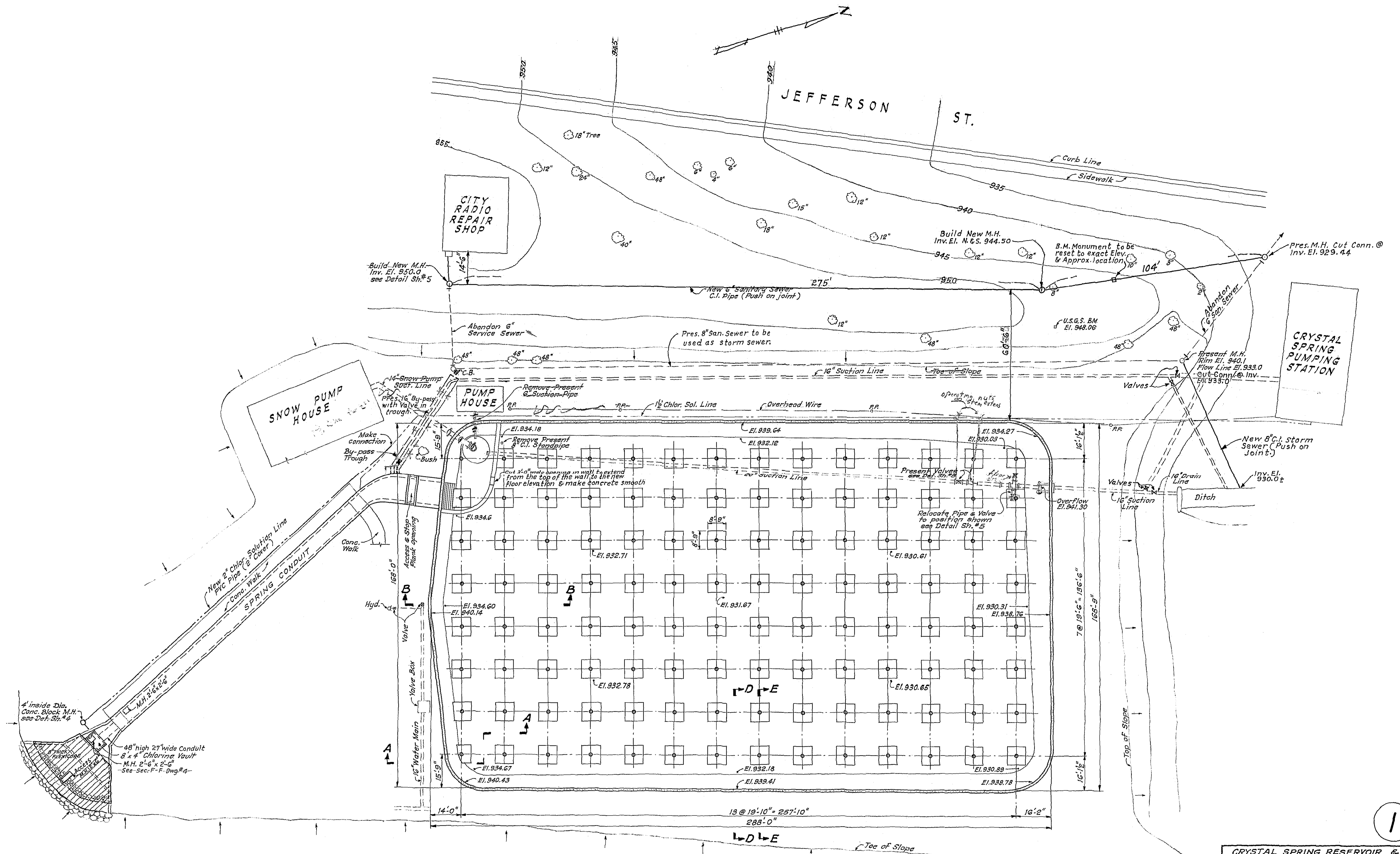
PLAN Scale: 1" = 20'-0"
