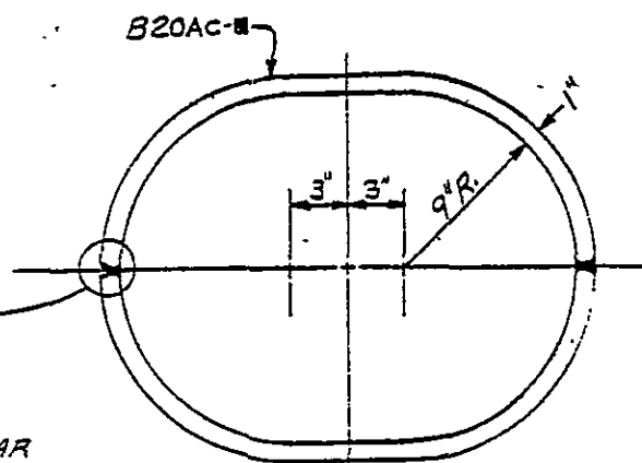
RING BAR DETAIL-MK. B20AC
