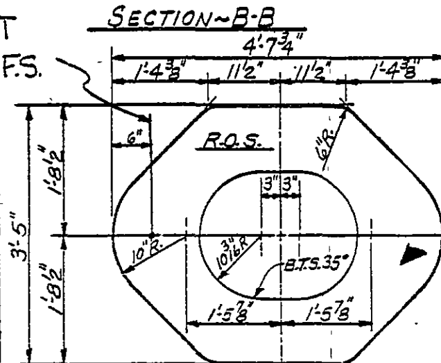
REINFORCING R. DETAIL-MK. B20Ae
