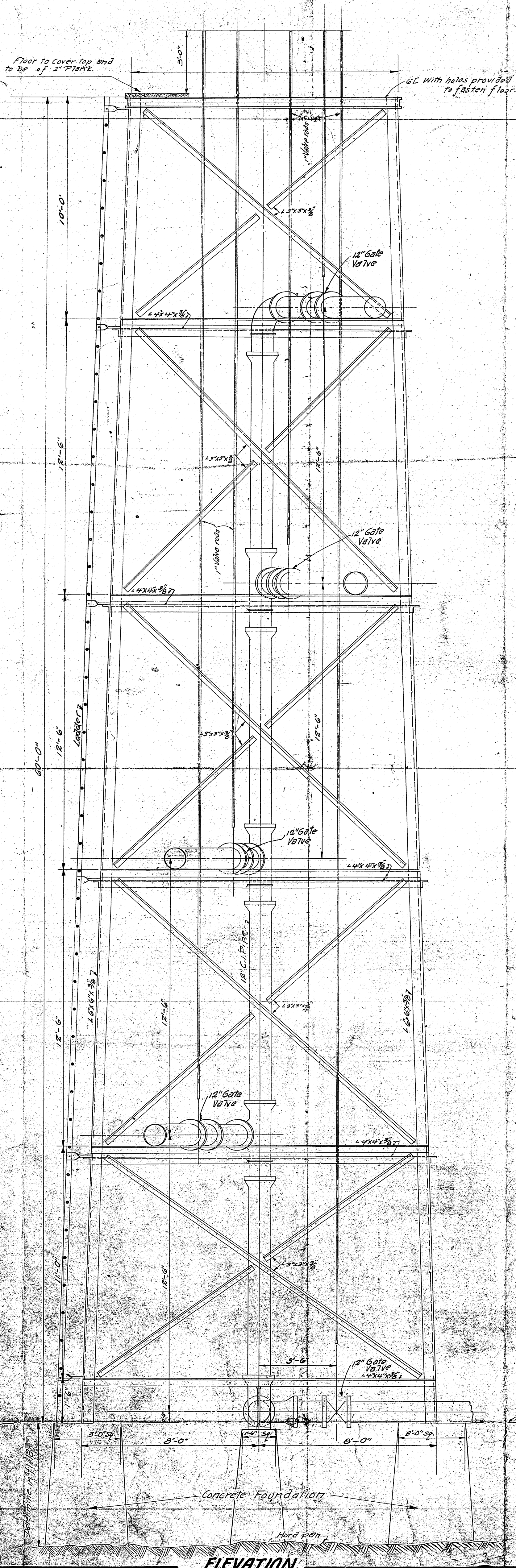
ELEVATION
