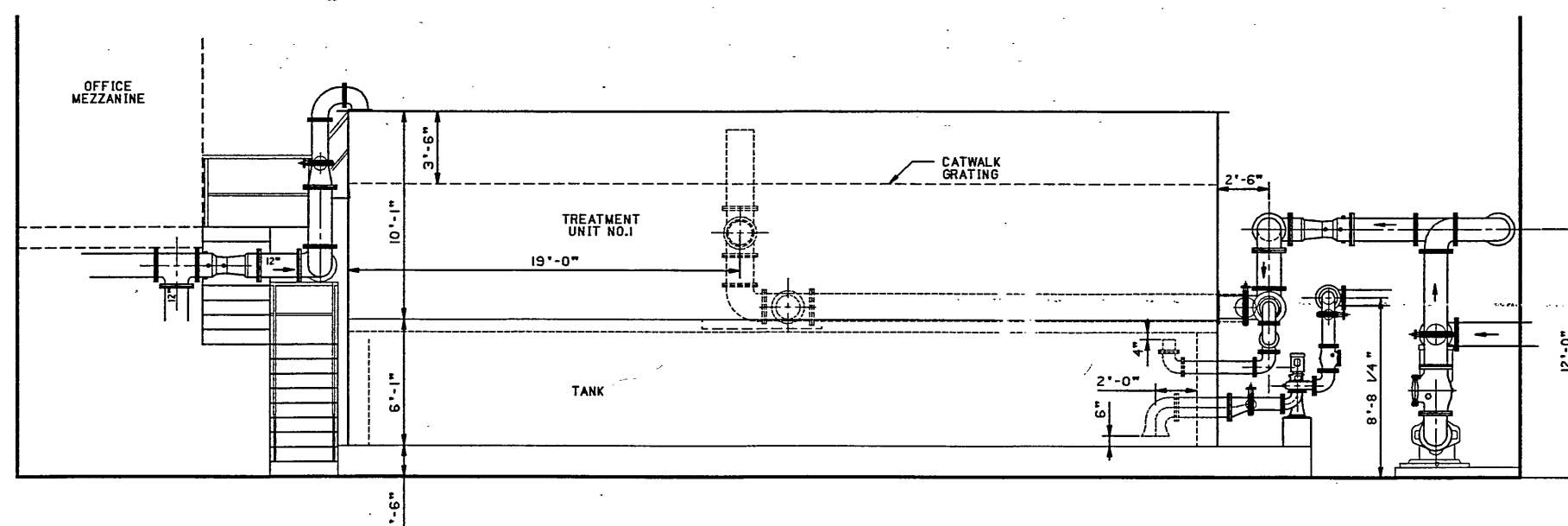
SECTION "A-A" SCALE: 1/4"=1'-0"
