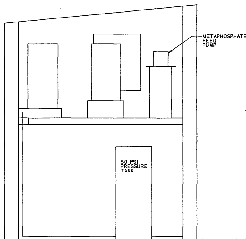
SECTION 2 SCALE: 1/2"=1'-0"
