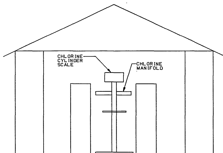
SECTION 1 SCALE: 1/2"=1'-0"
