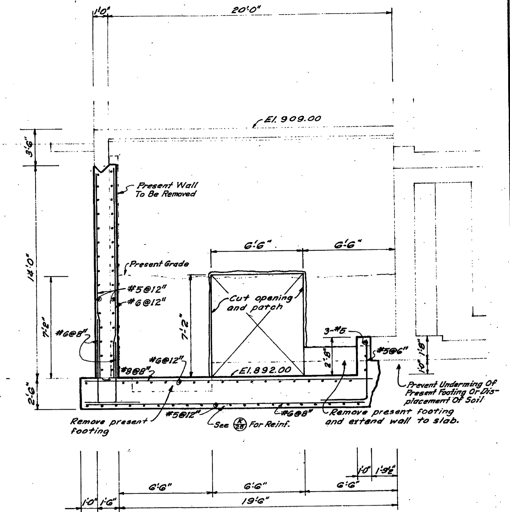
SECTION E 18-19 Scale: 4"=1'-0"
