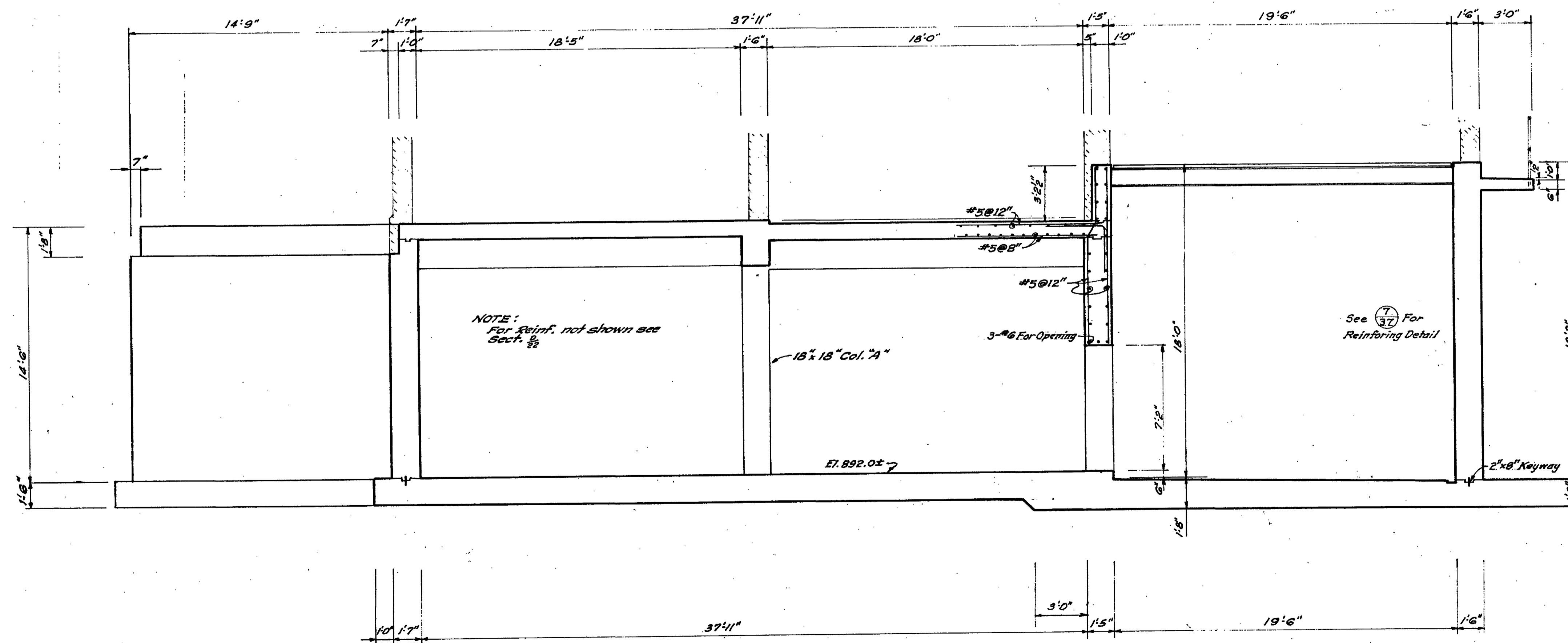
SECTION F 18-19 Scale: 4"=1'-0"
