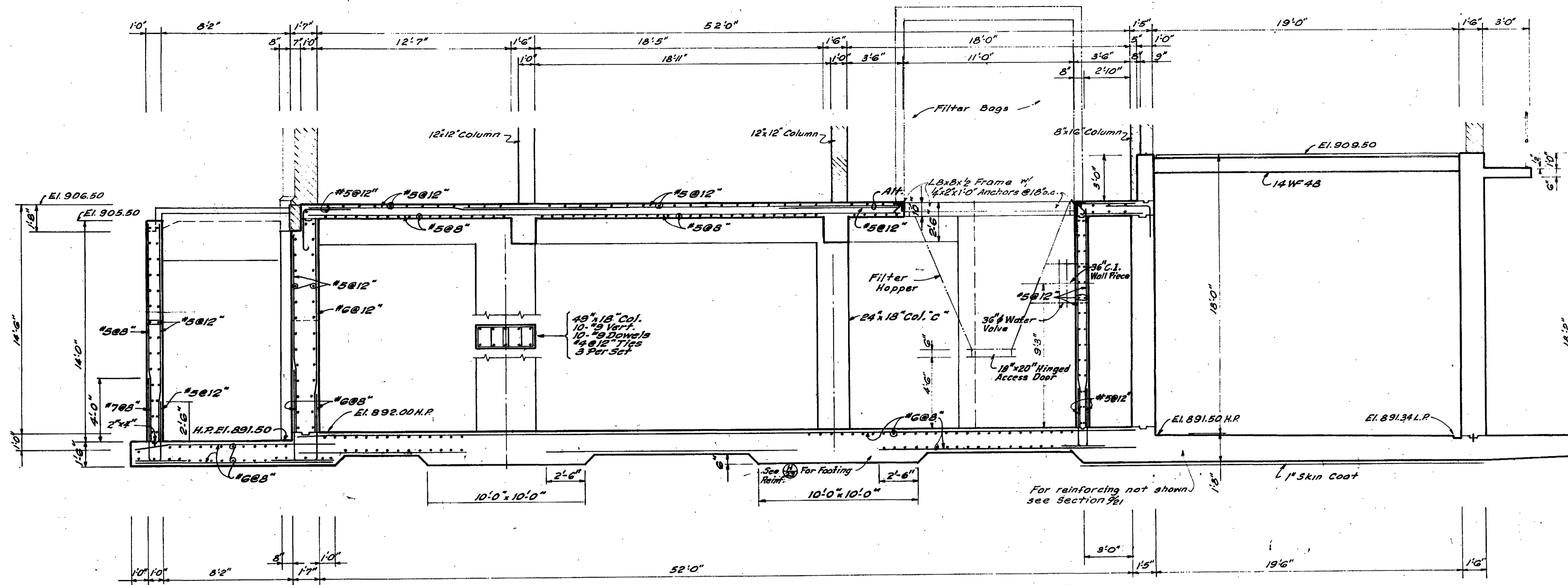
SECTION D 18-19 Scale: 4"=1'-0"
