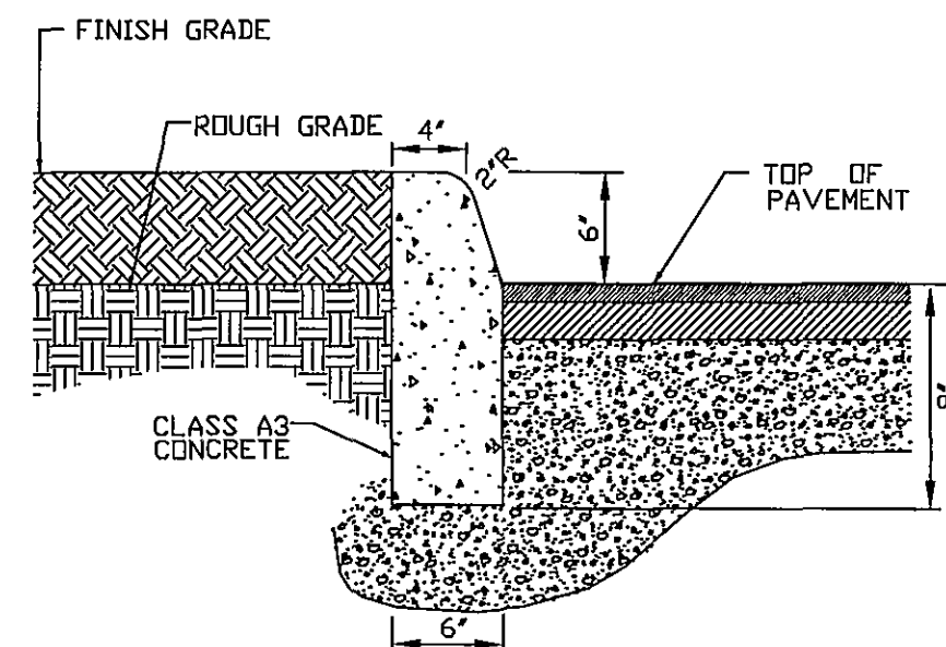
CG-2 DETAIL N.T.S.
