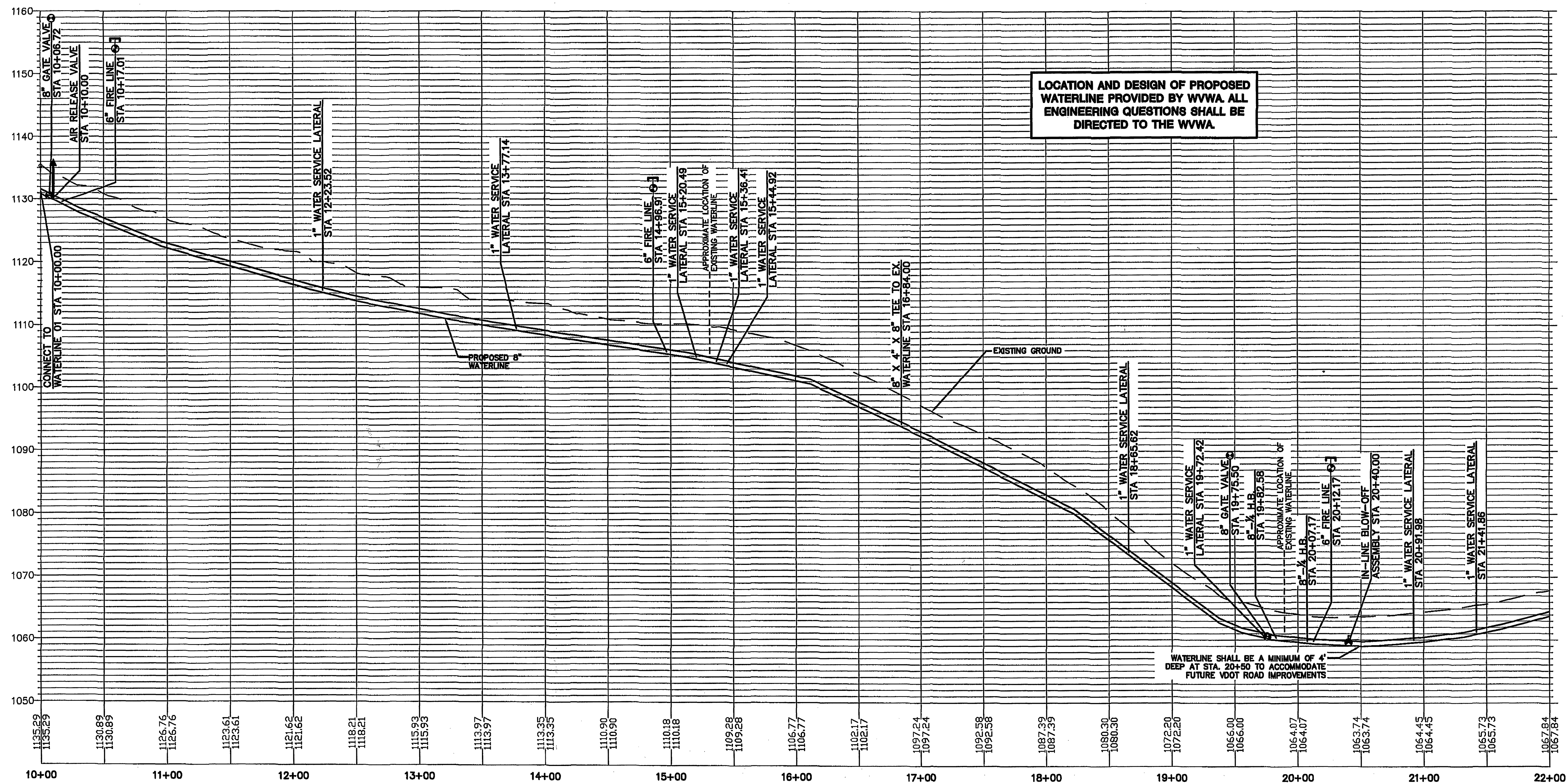
HUFFMAN LN. STA 10+00.00 TO STA 22+00.00 PROFILE
