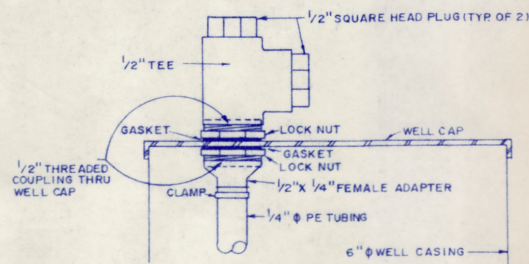
WELL CAP DETAIL N.T.S.
