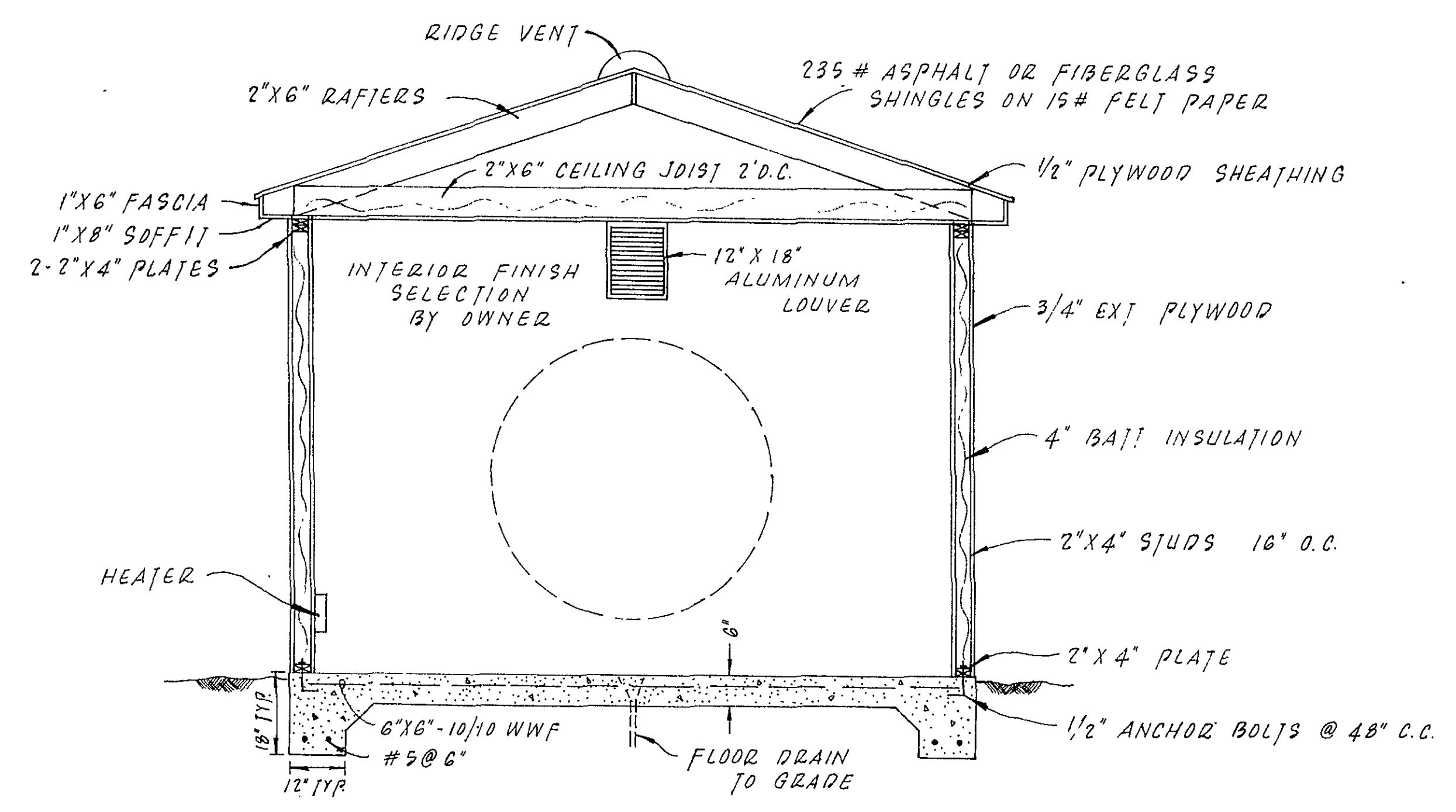
SECTION A-A
