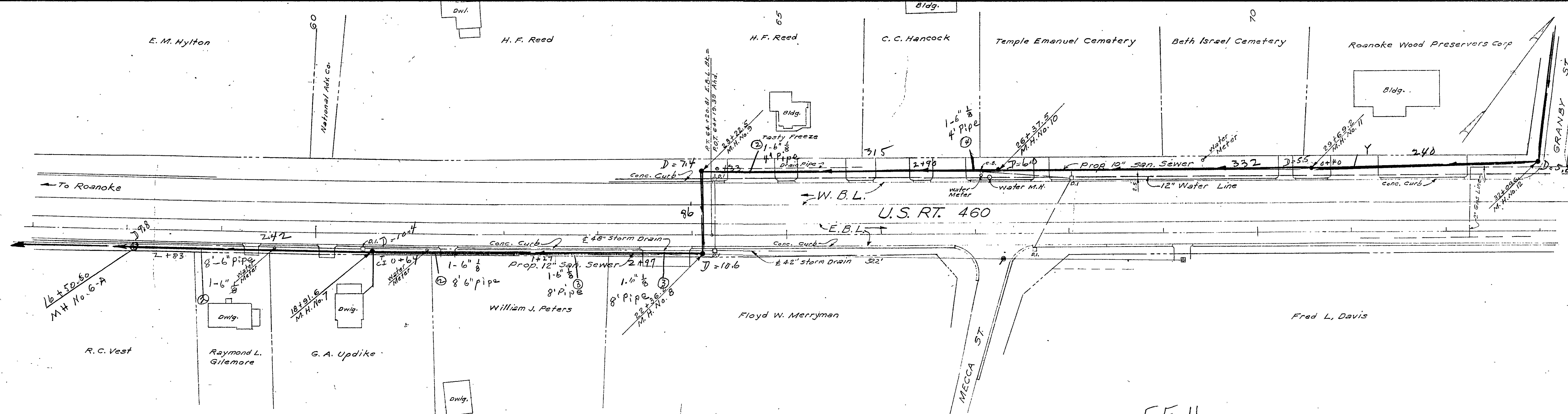
PLAN Scale: 1" = 50'
