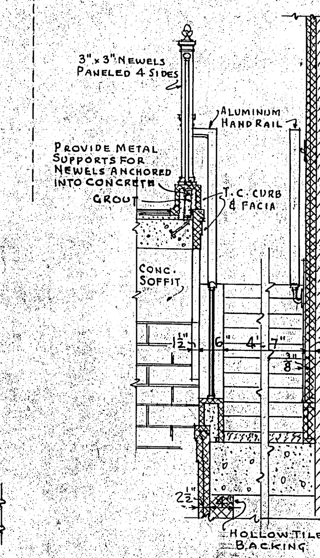
SECTION A-A
