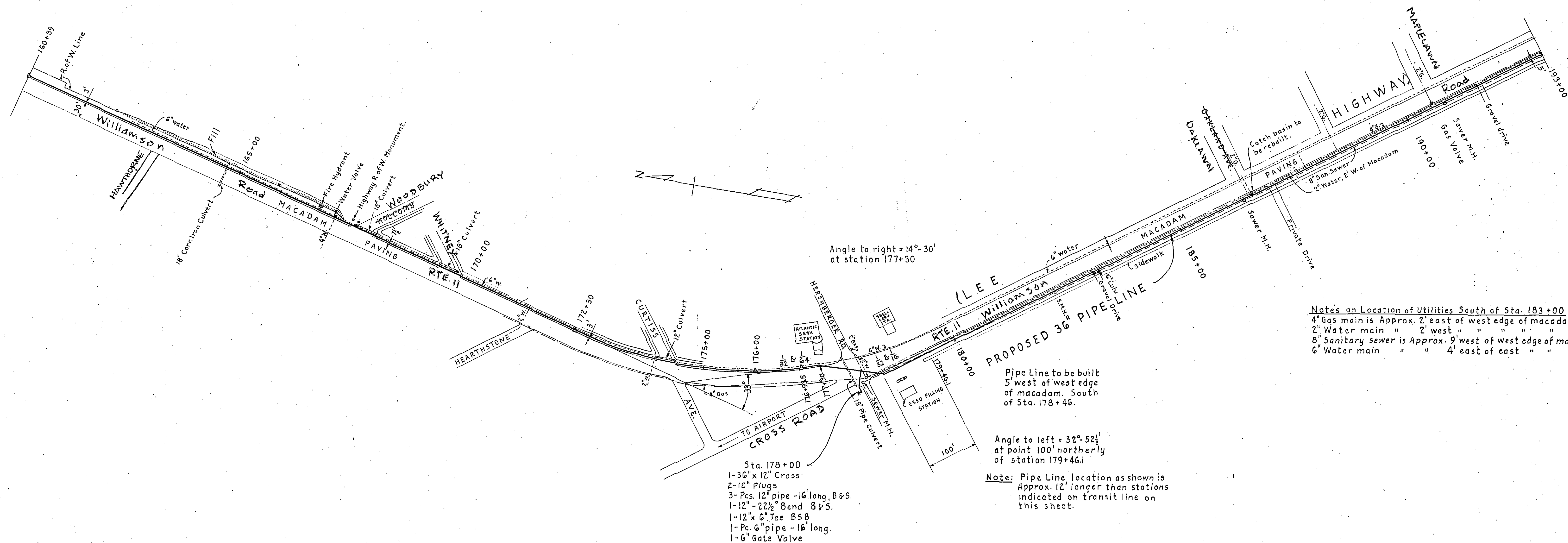
PLAN - STA. 160+39 to 193+00
