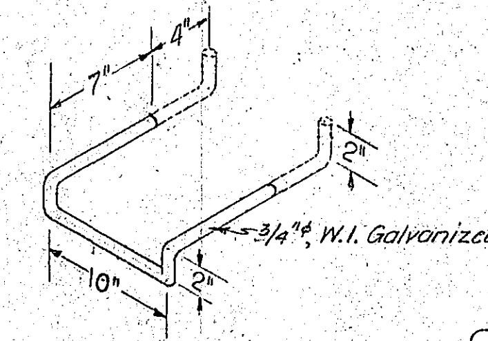
MANHOLE STEP SCALE: 1 1/2" = 1'-0"
