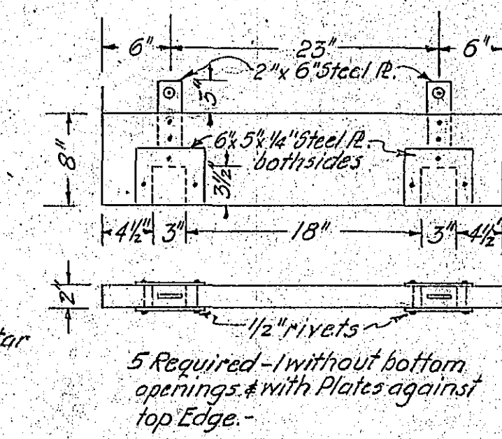
STOP LOG SCALE: 1" = 1'-0"
