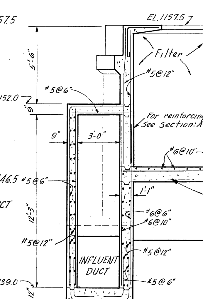
SECTION-G-G Scale: \frac{1}{4}'' = 1'-0''
