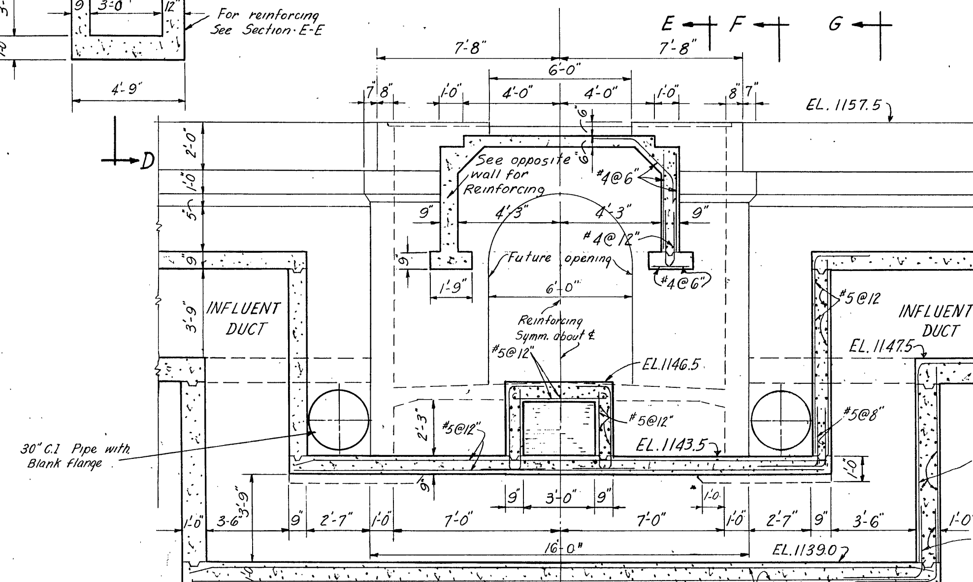
SECTION-D-D Scale: \frac{1}{4}'' = 1'-0''
