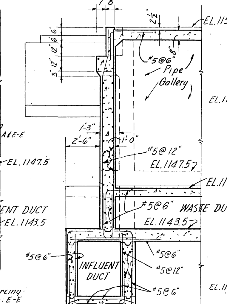
SECTION-E-E Scale: \frac{1}{4}'' = 1'-0''
