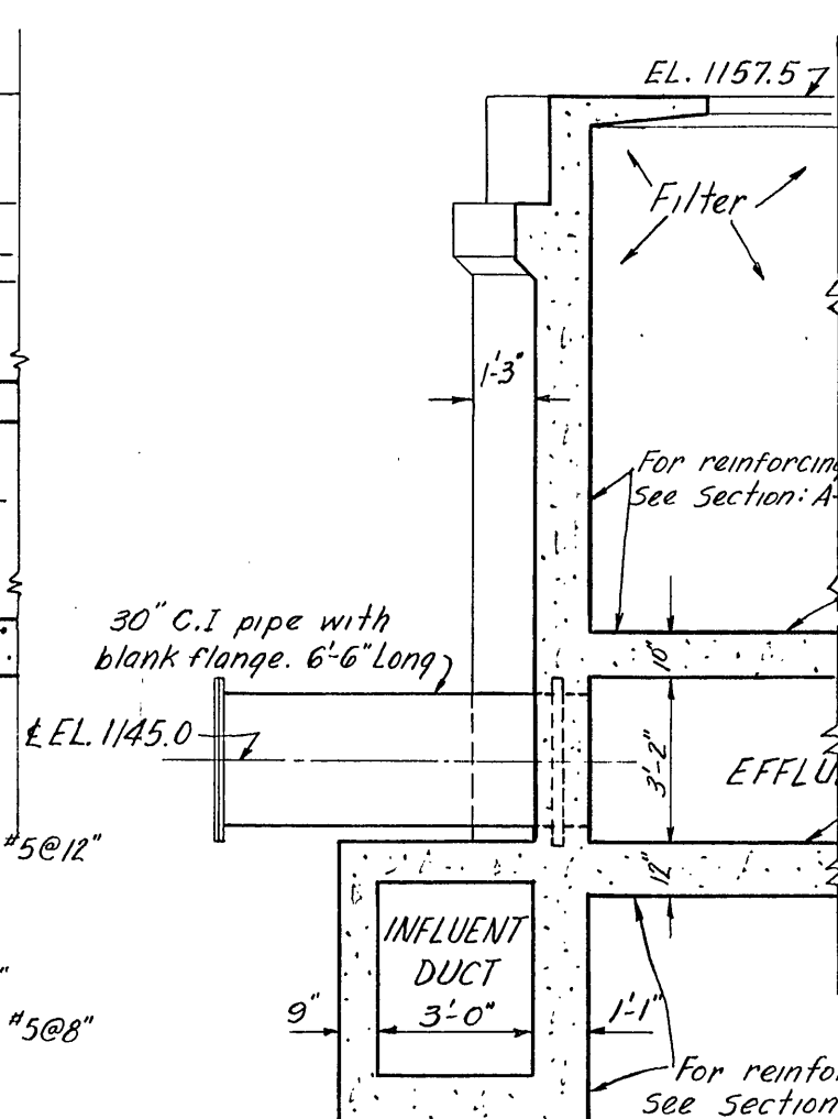
SECTION-F-F Scale: \frac{1}{4}'' = 1'-0''
