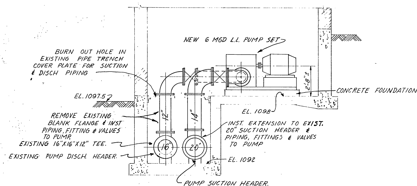
SECTION: A-A SCALE: \frac{1}{4}" = 1'-0"
