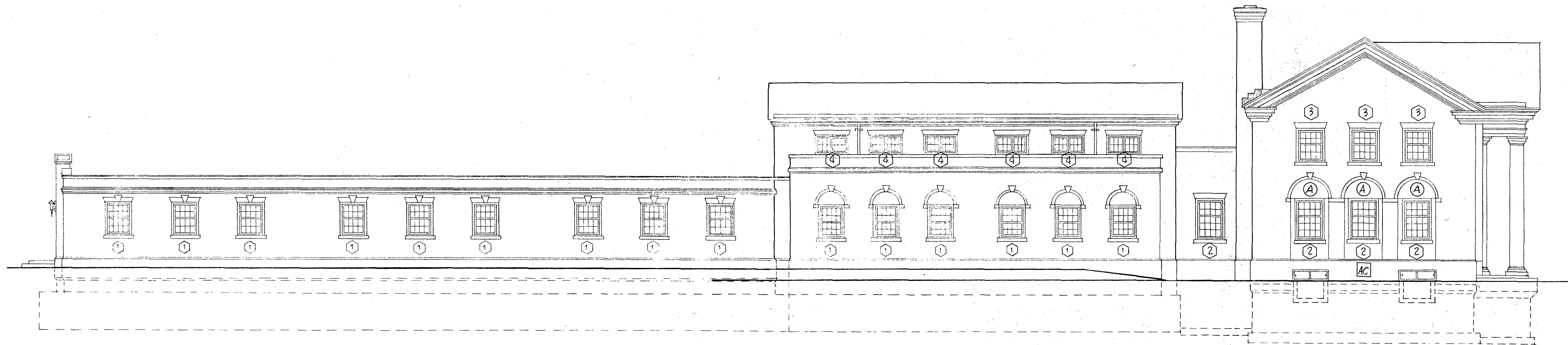
LEFT ELEVATION SCALE: 1/8" = 1' 0"
