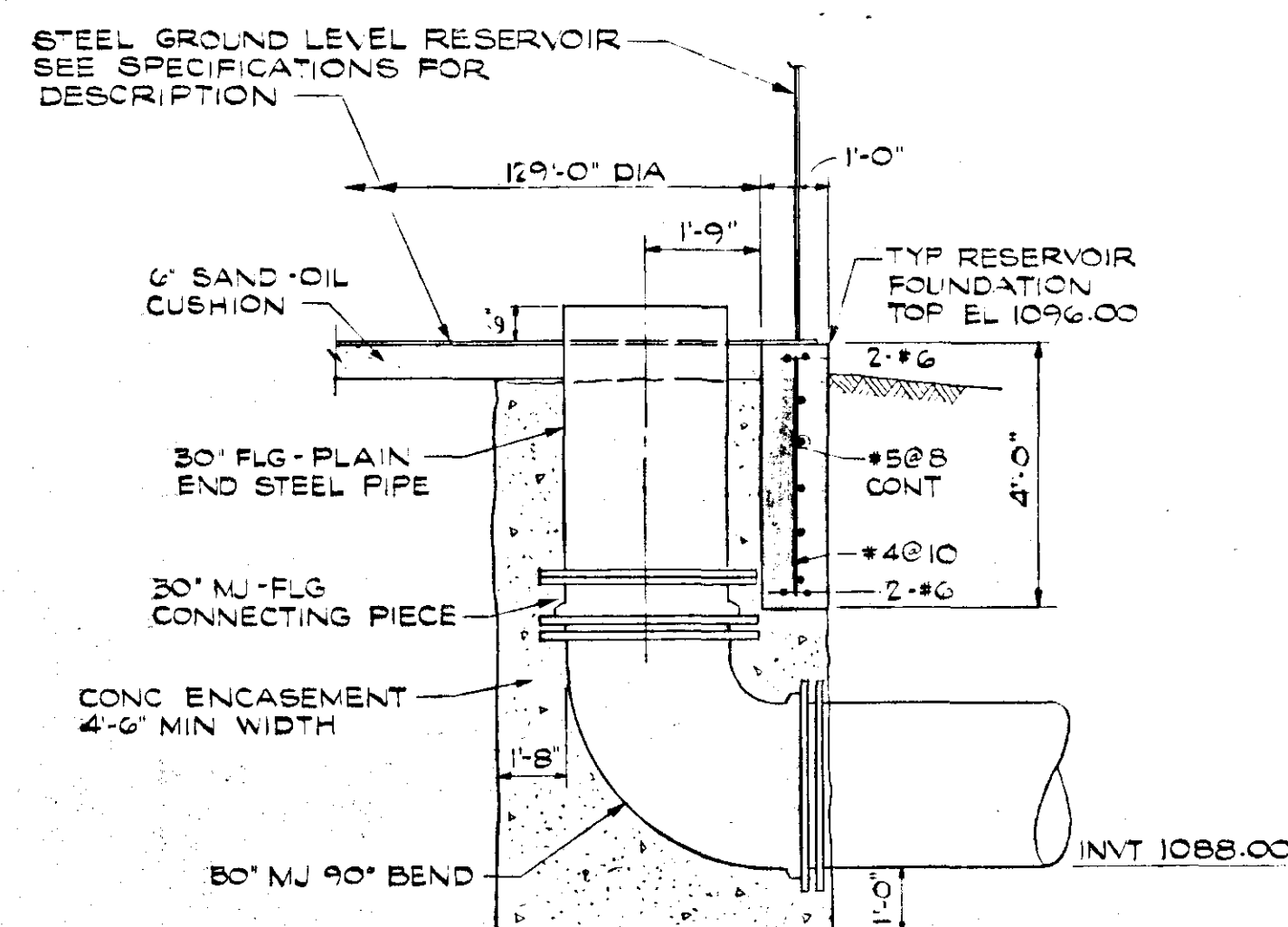
SECTION C1.2 SCALE: 3/8" = 1'-0"
