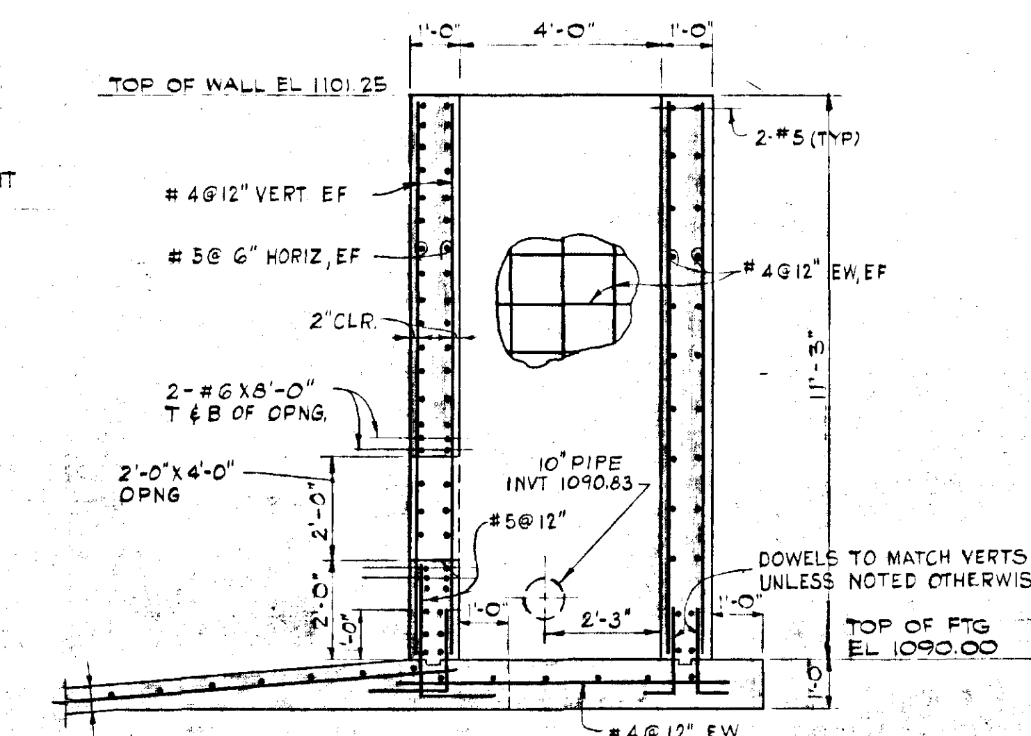
SECTION C9.5 SCALE: 3/8" = 1'-0" C9
