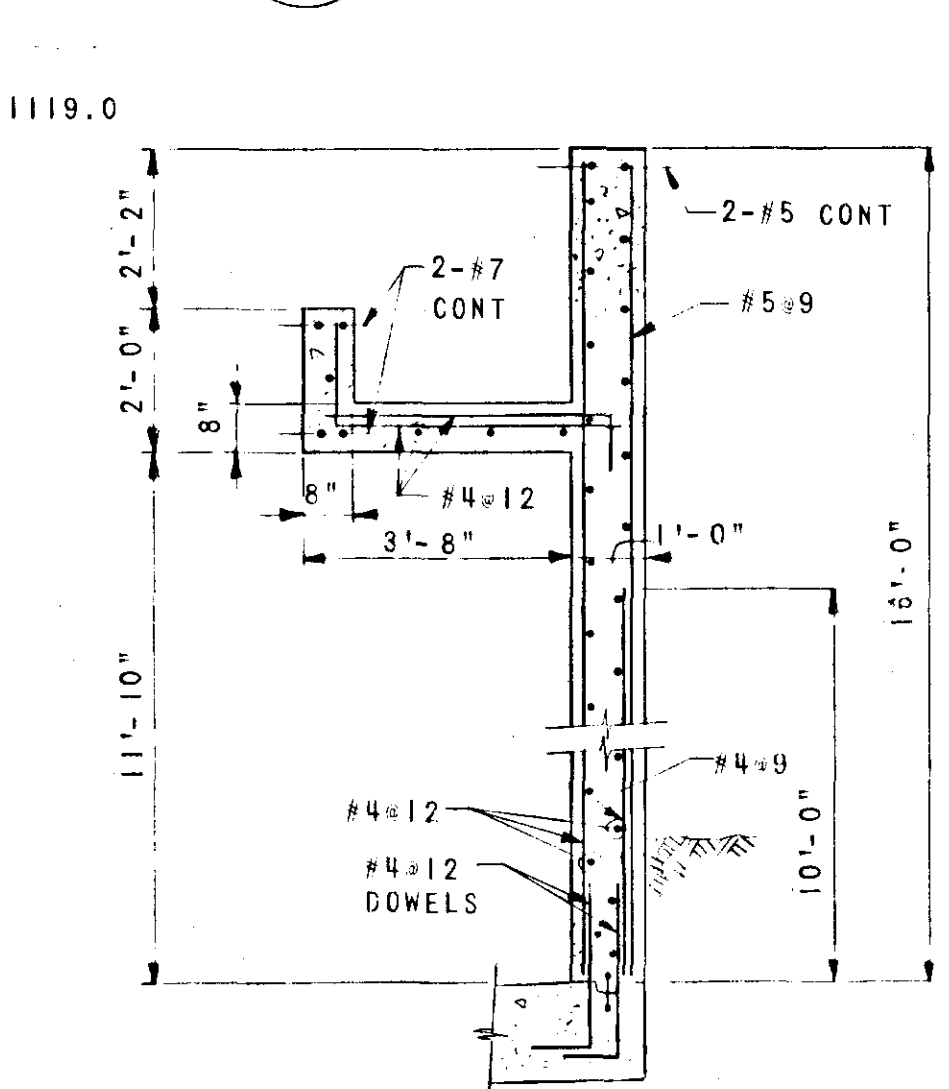
SECTION SCALE: \frac{3}{8} "=1'-0"
