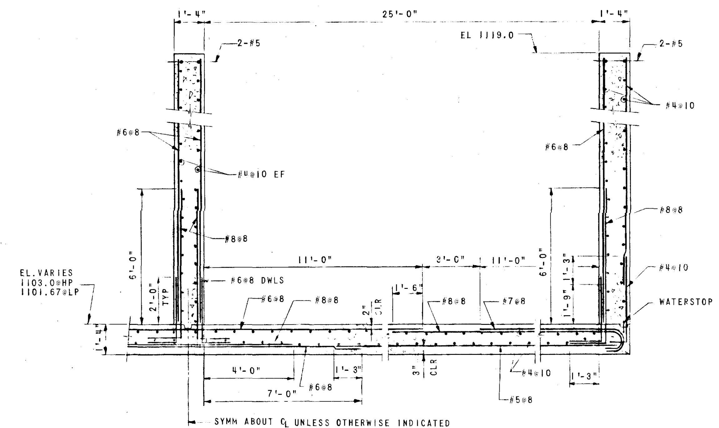
SECTION SCALE: \frac{3}{8} "=1'-0"
