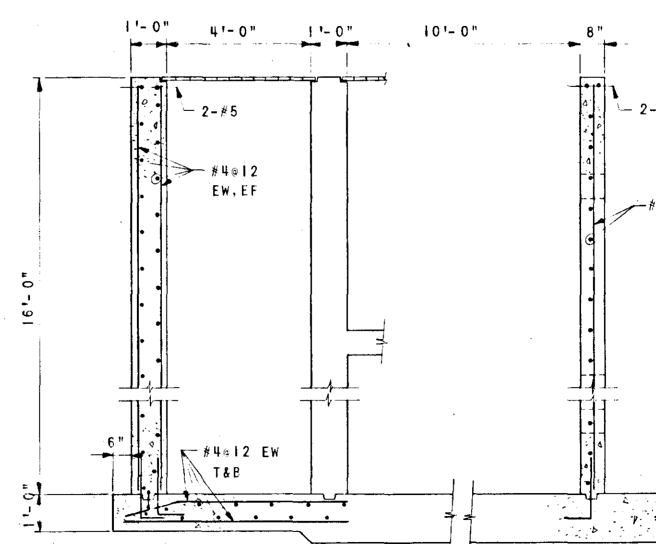
SECTION SCALE: \frac{3}{8} "=1'-0"
