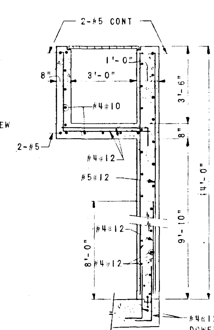
SECTION SCALE: \frac{3}{8} "=1'-0"
