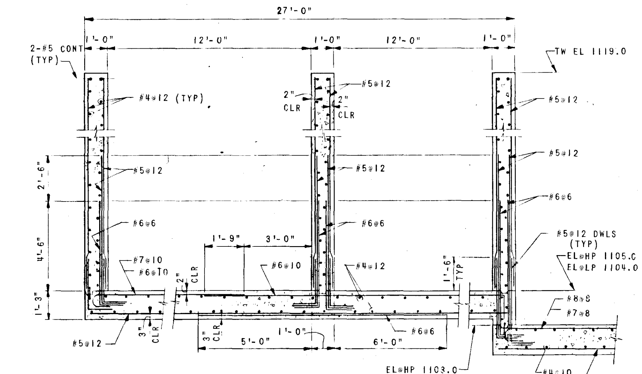
SECTION SCALE: \frac{3}{8} "=1'-0"
